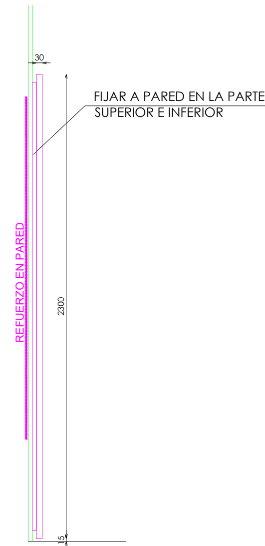
PERFIL
