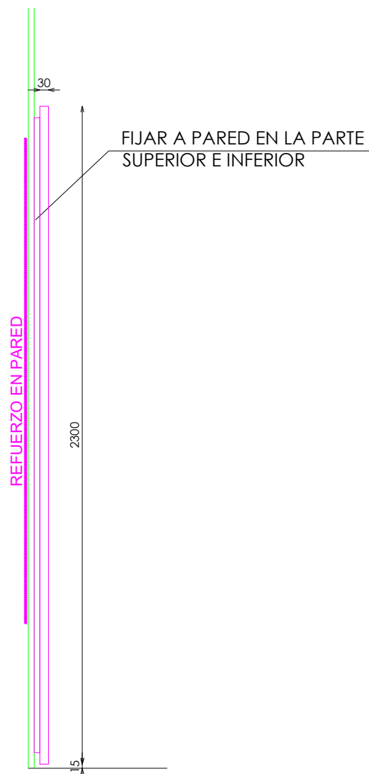
PERFIL
