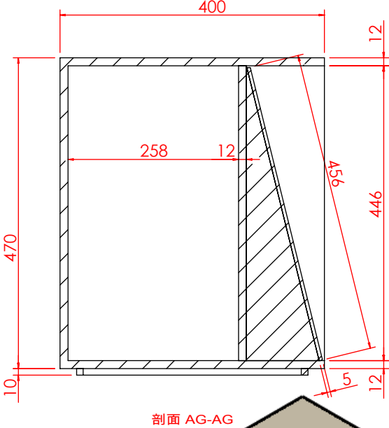
剖面 AG-AG
