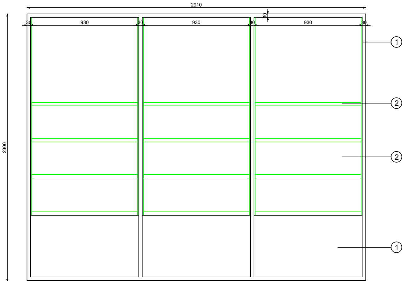
ALZADO FRONTAL
