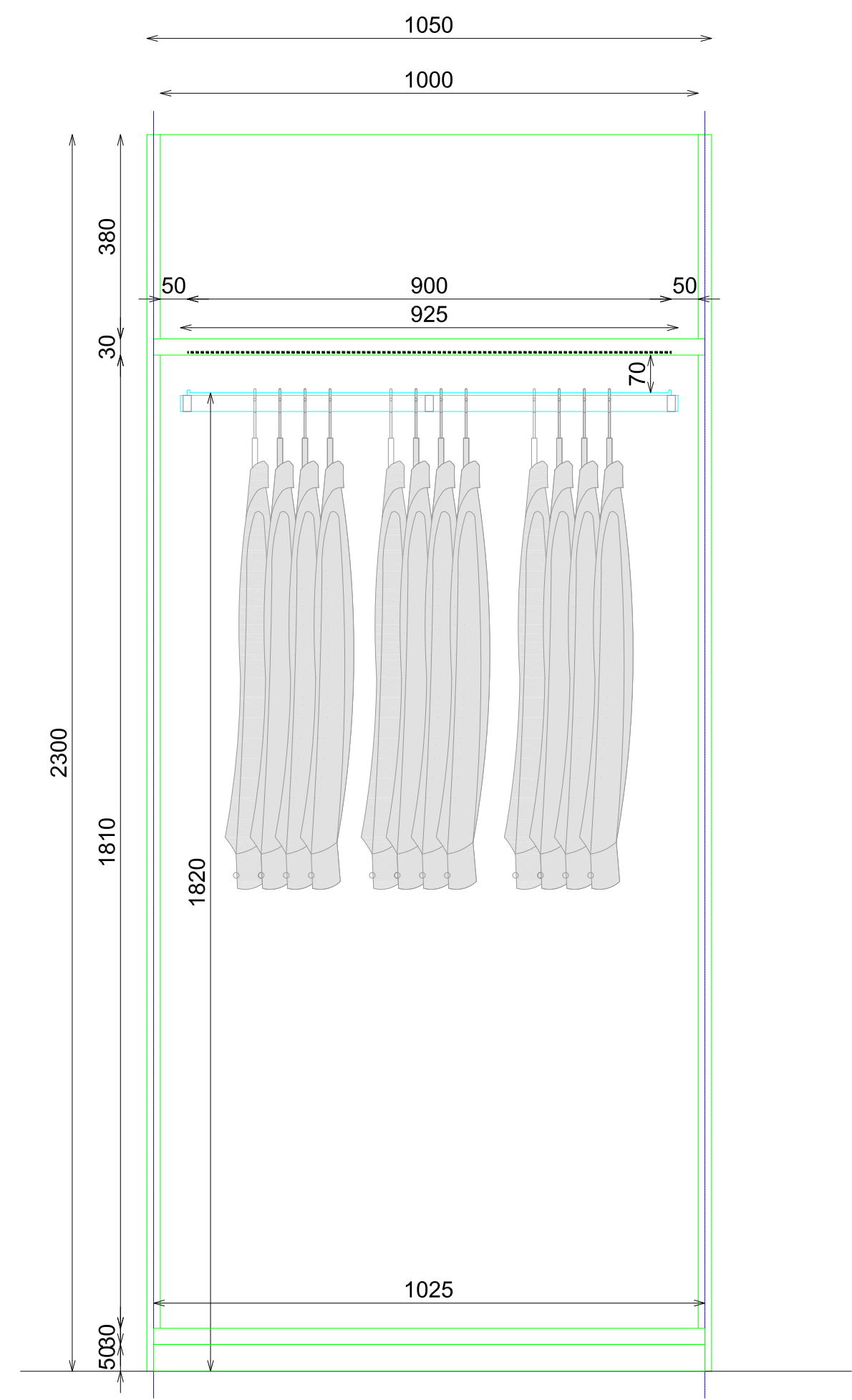
ALZADO
