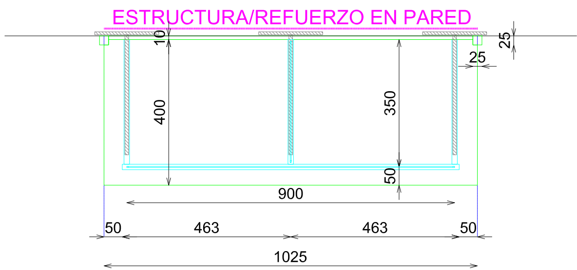
PLANTA
