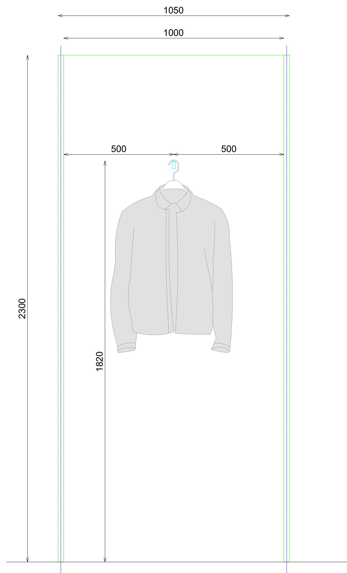
ALZADO
