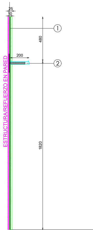
SECCION
