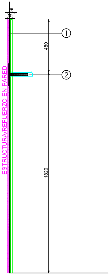
SECCION
