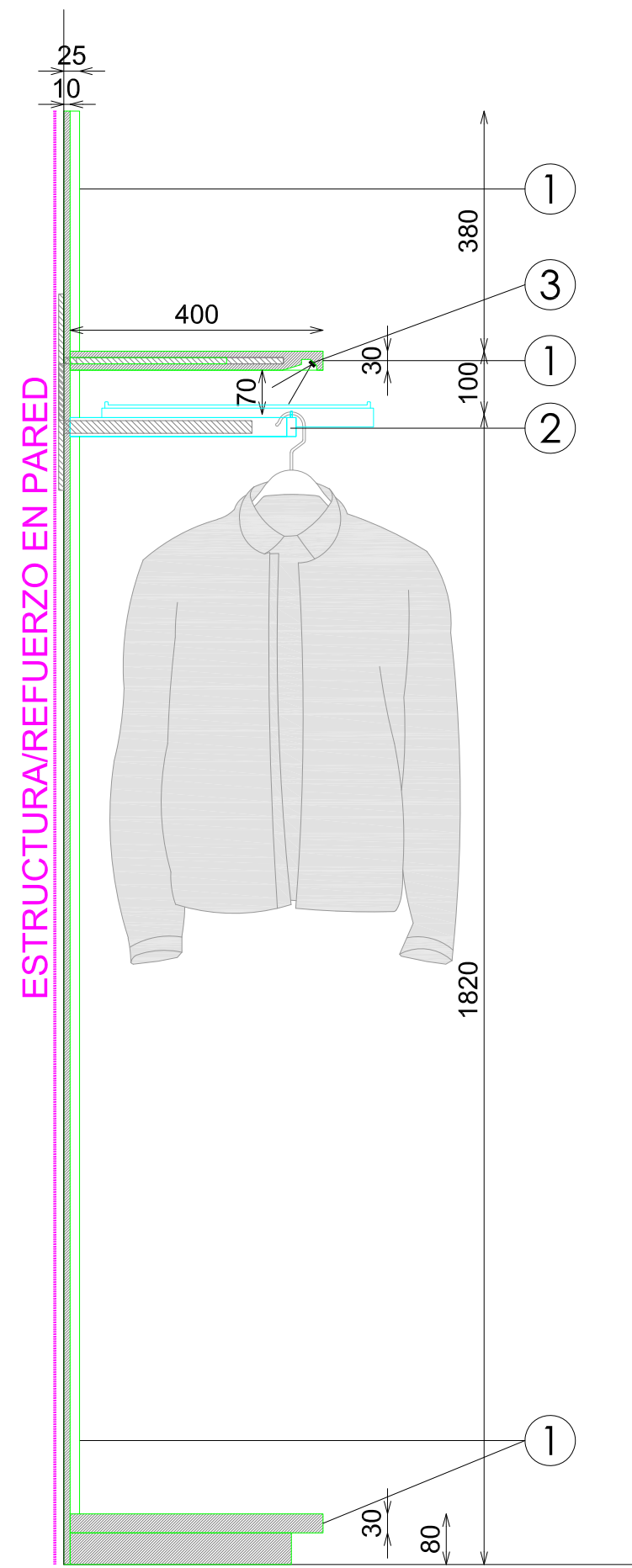
SECCION
