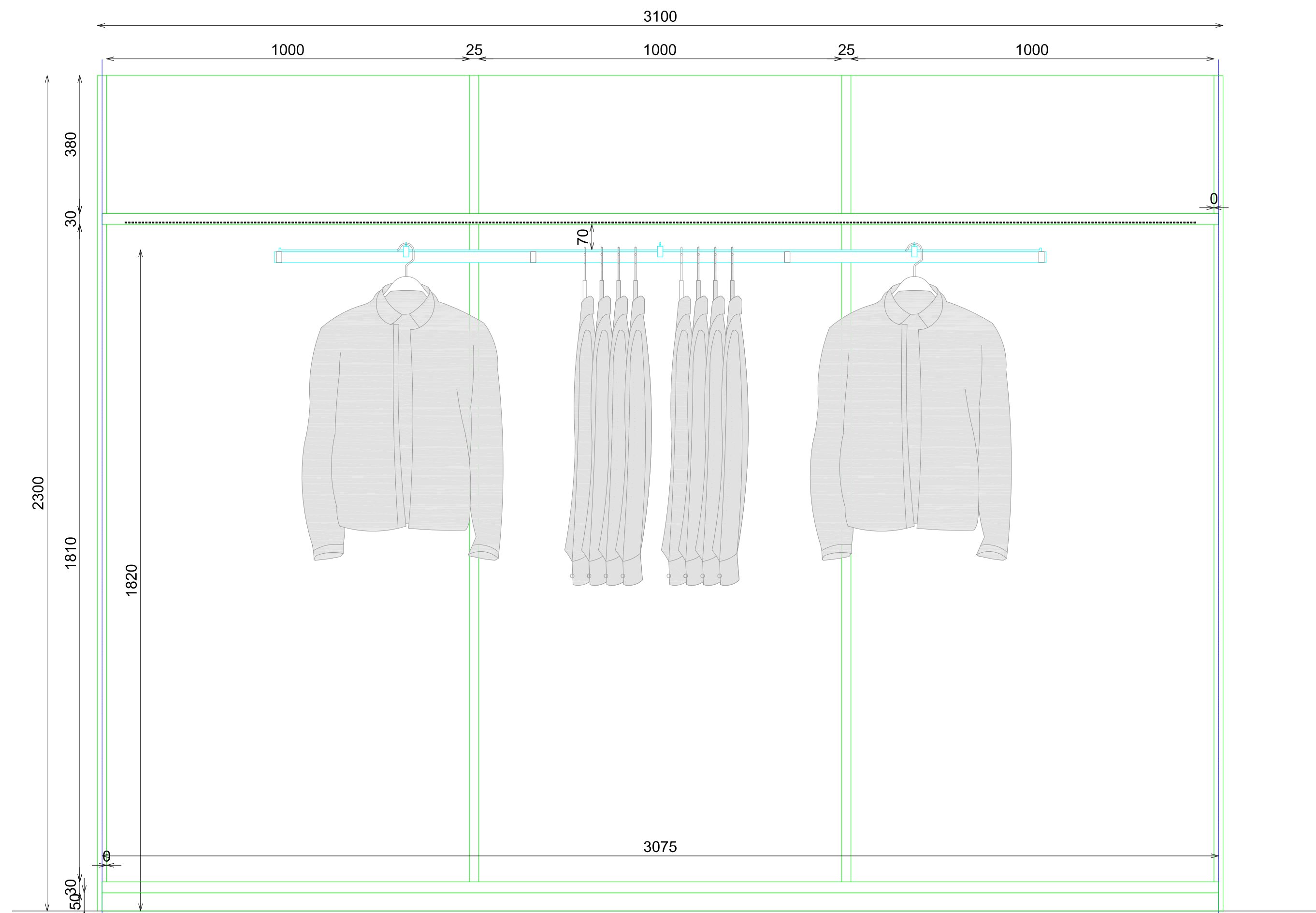
ALZADO
