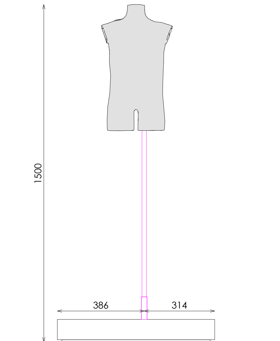
PERFIL
