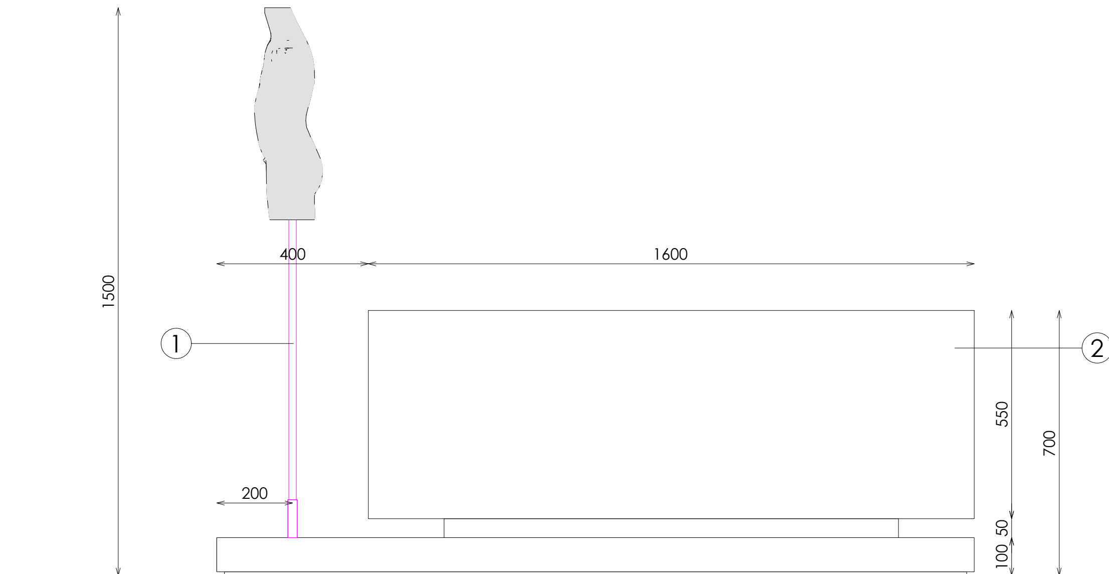
ALZADO
