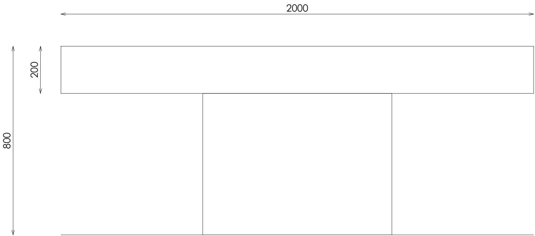
ALZADO
