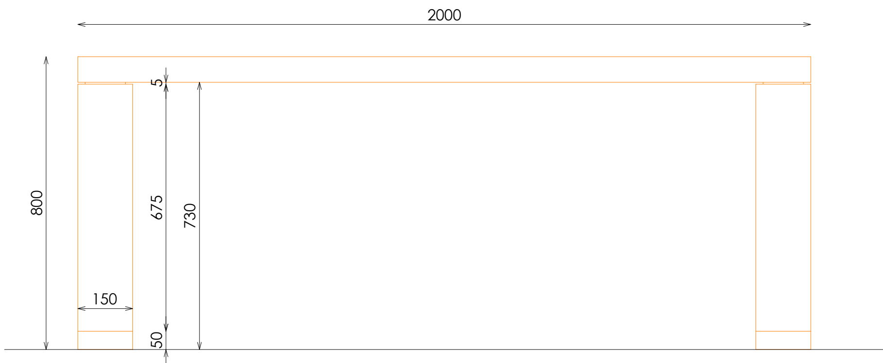
ALZADO
