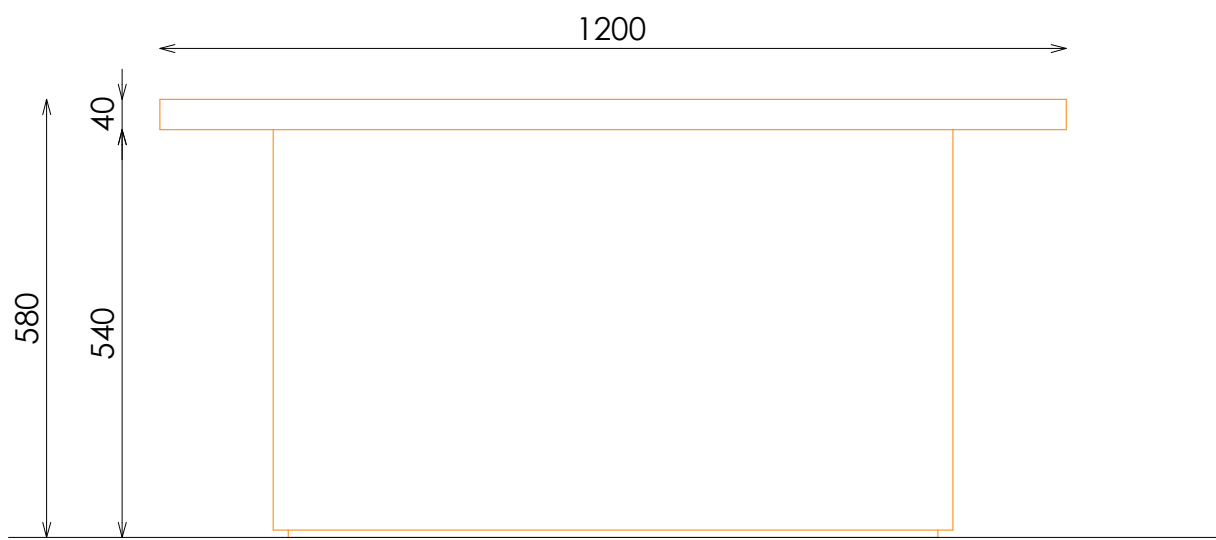
ALZADO
