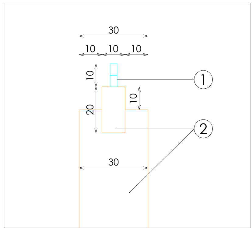
DETALLE A
