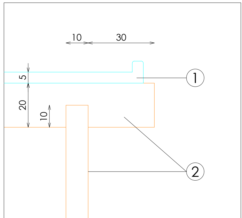
DETALLE B
