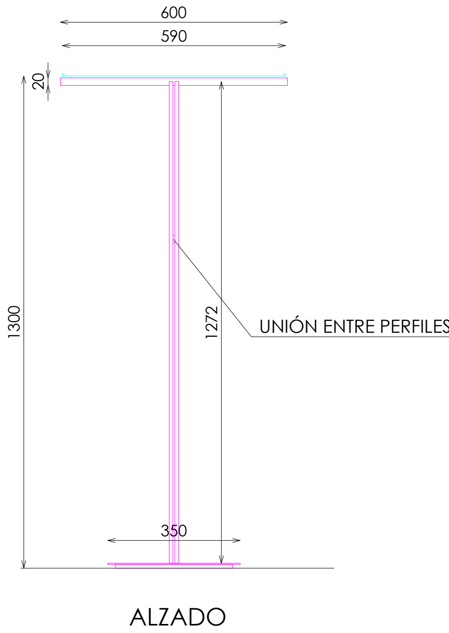
ALZADO
