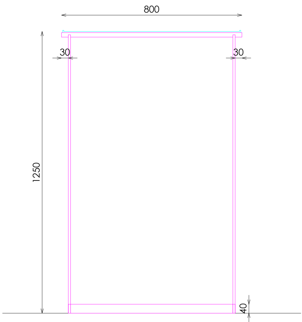
ALZADO
