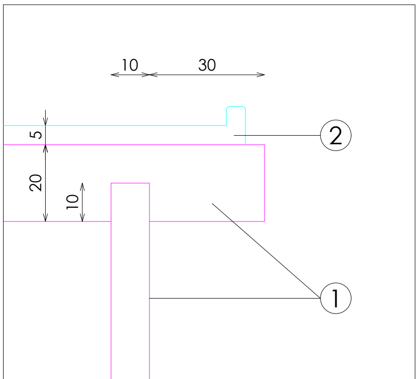
DETALLE B
