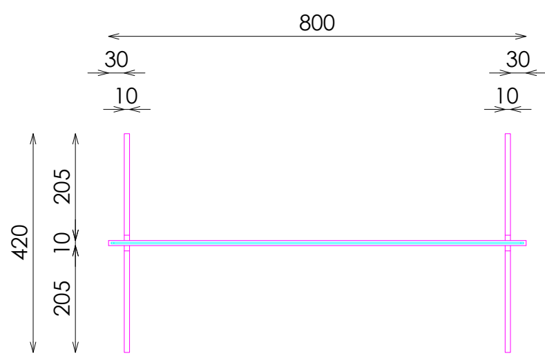
PLANTA
