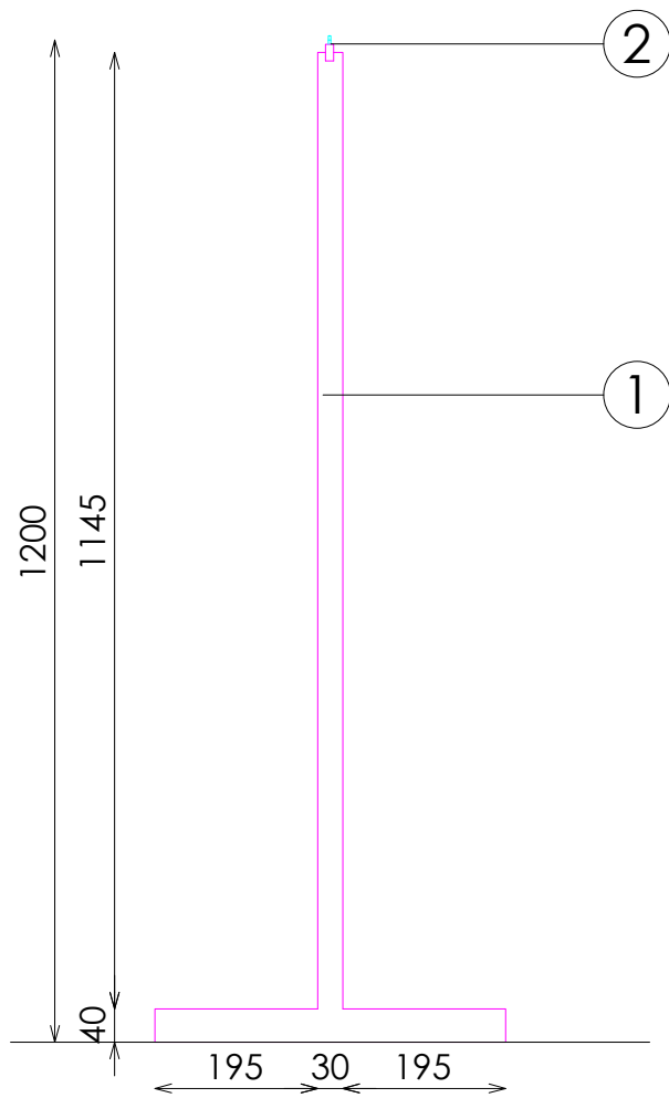
SECCIÓN
