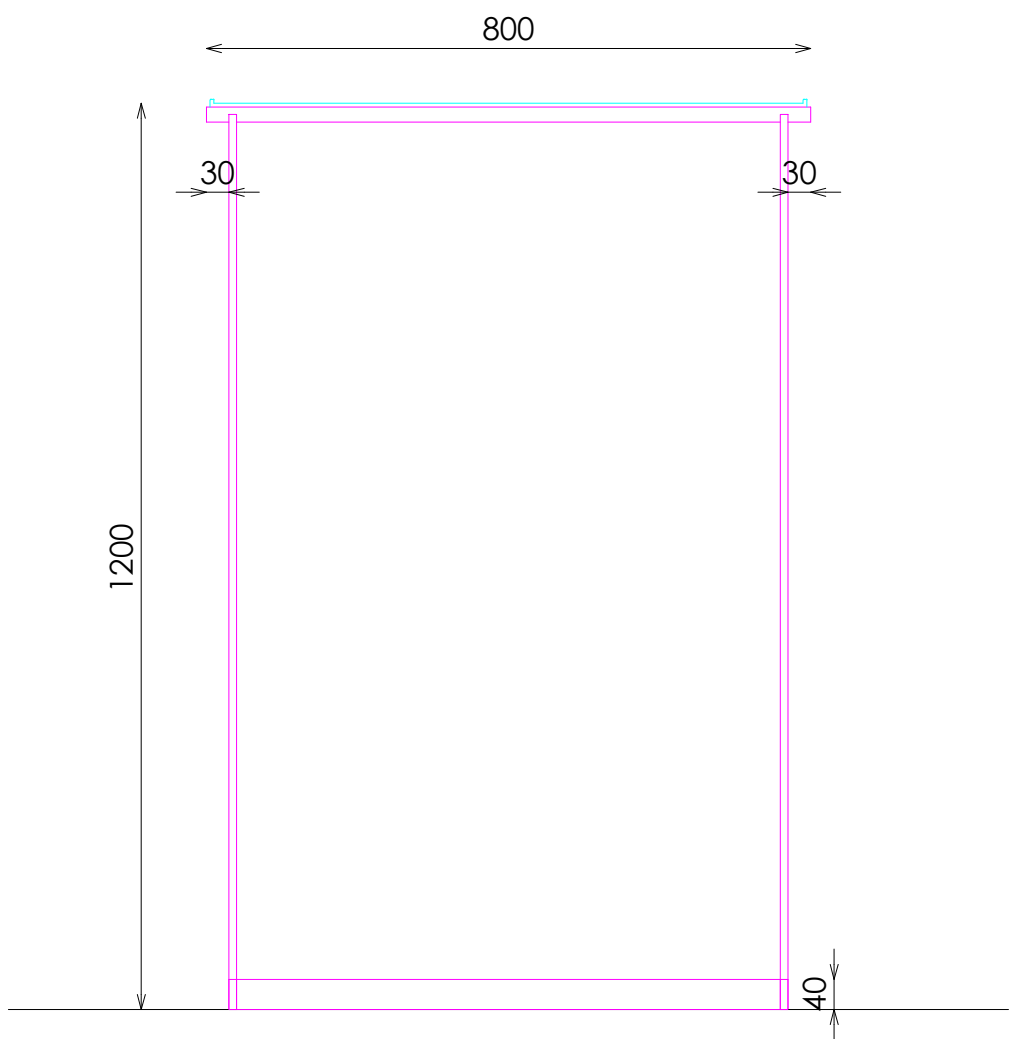
ALZADO
