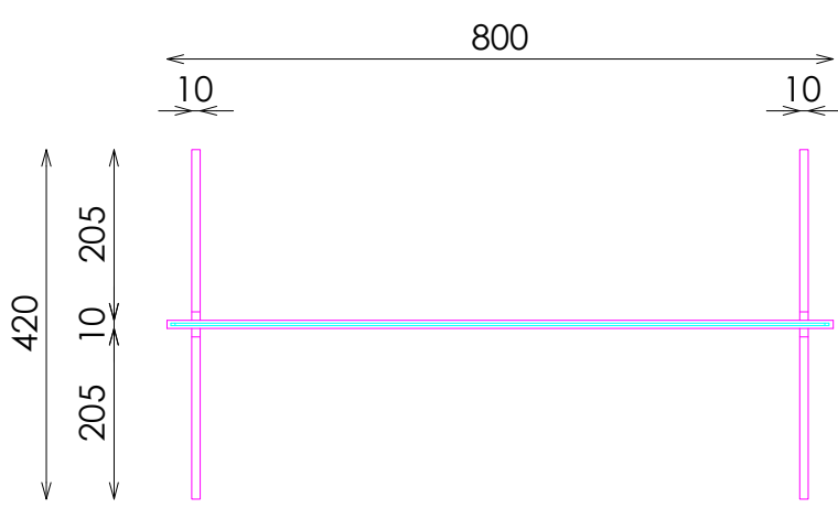
PLANTA
