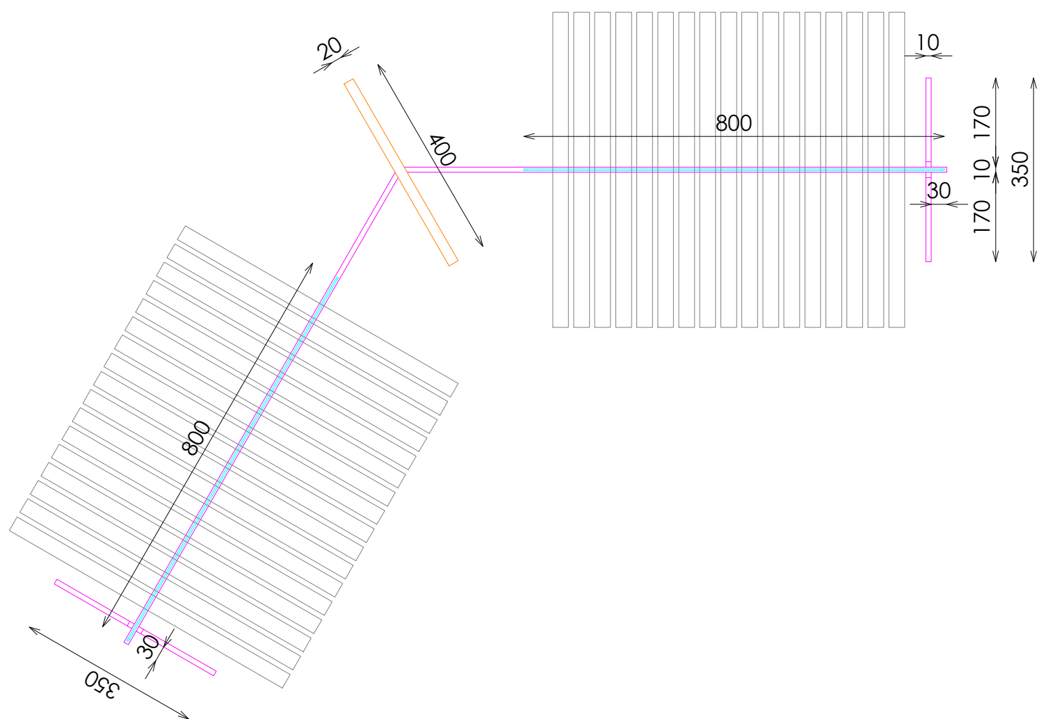
PLANTA
