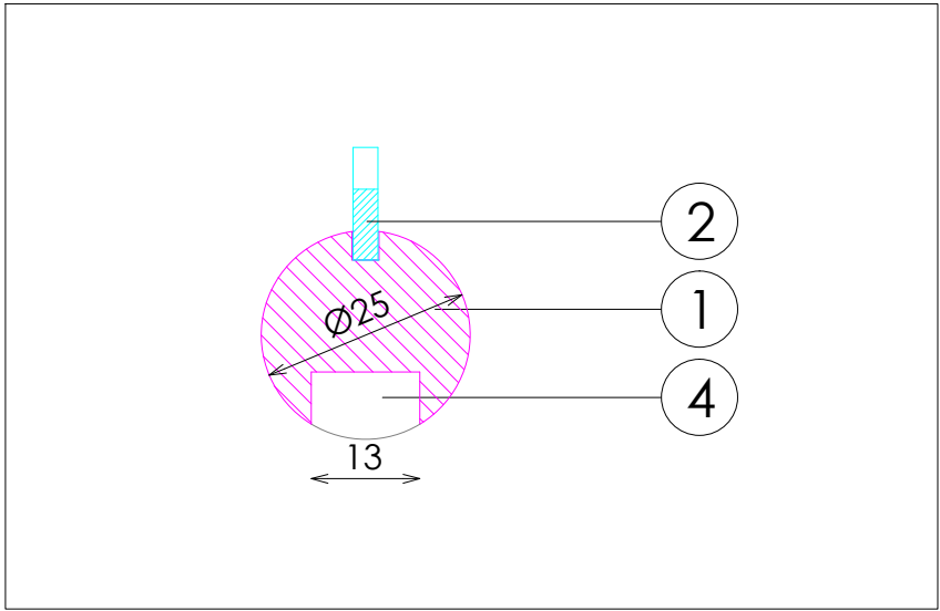
DETALLE A
