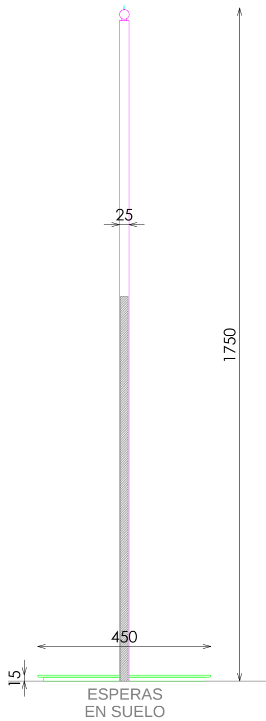
SECCION
