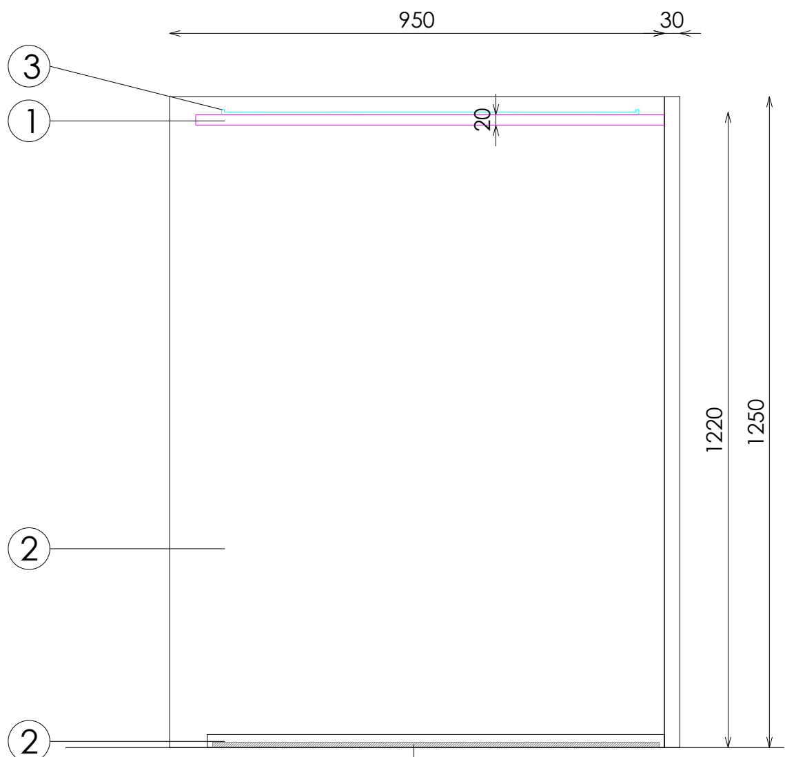
ALZADO
