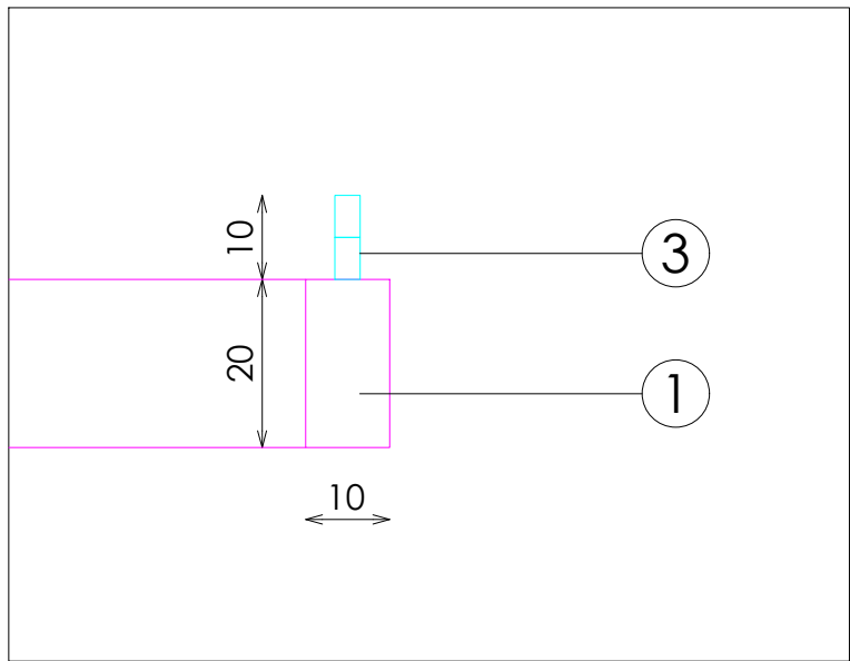
DETALLE B
