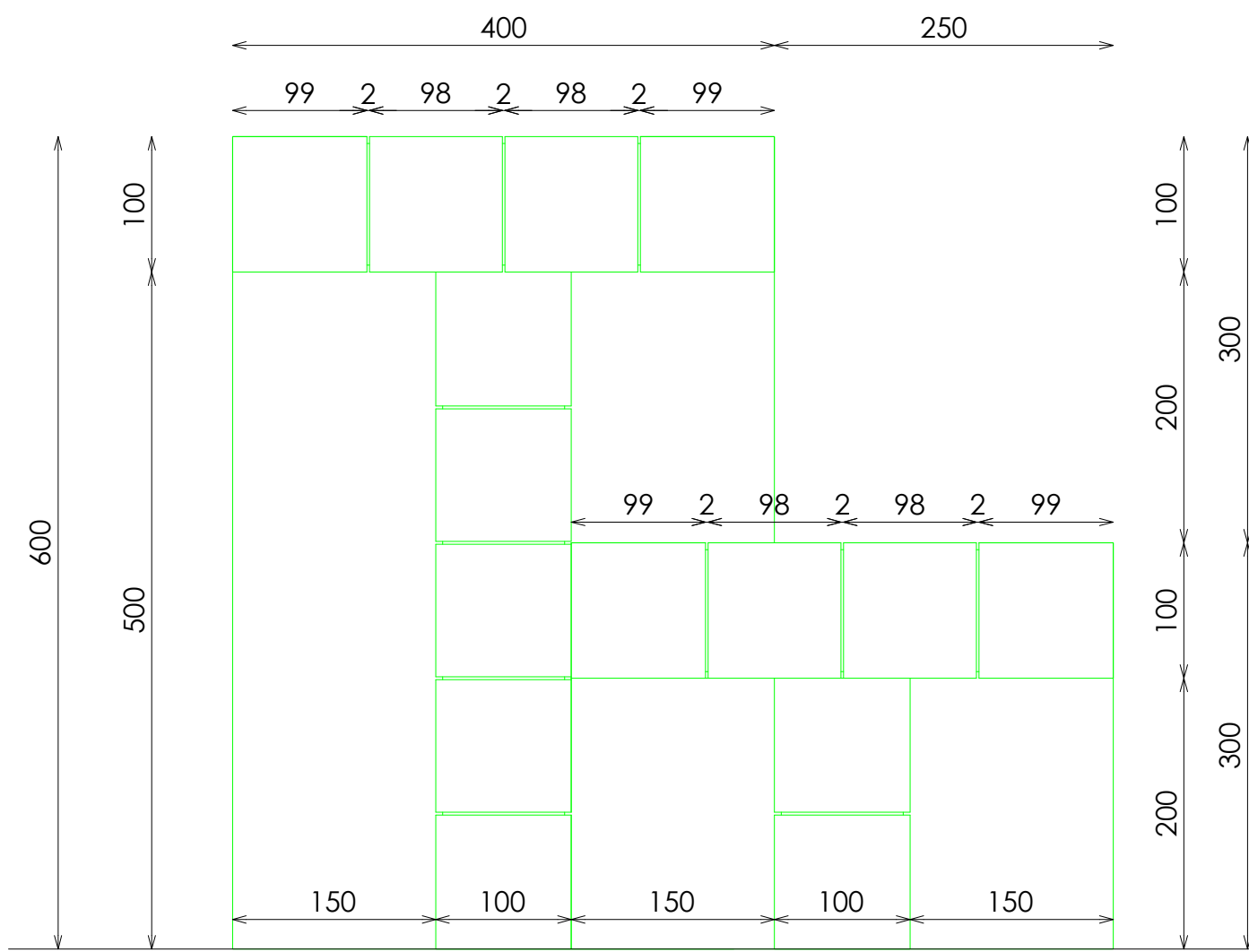
ALZADO IZQUIERDO
