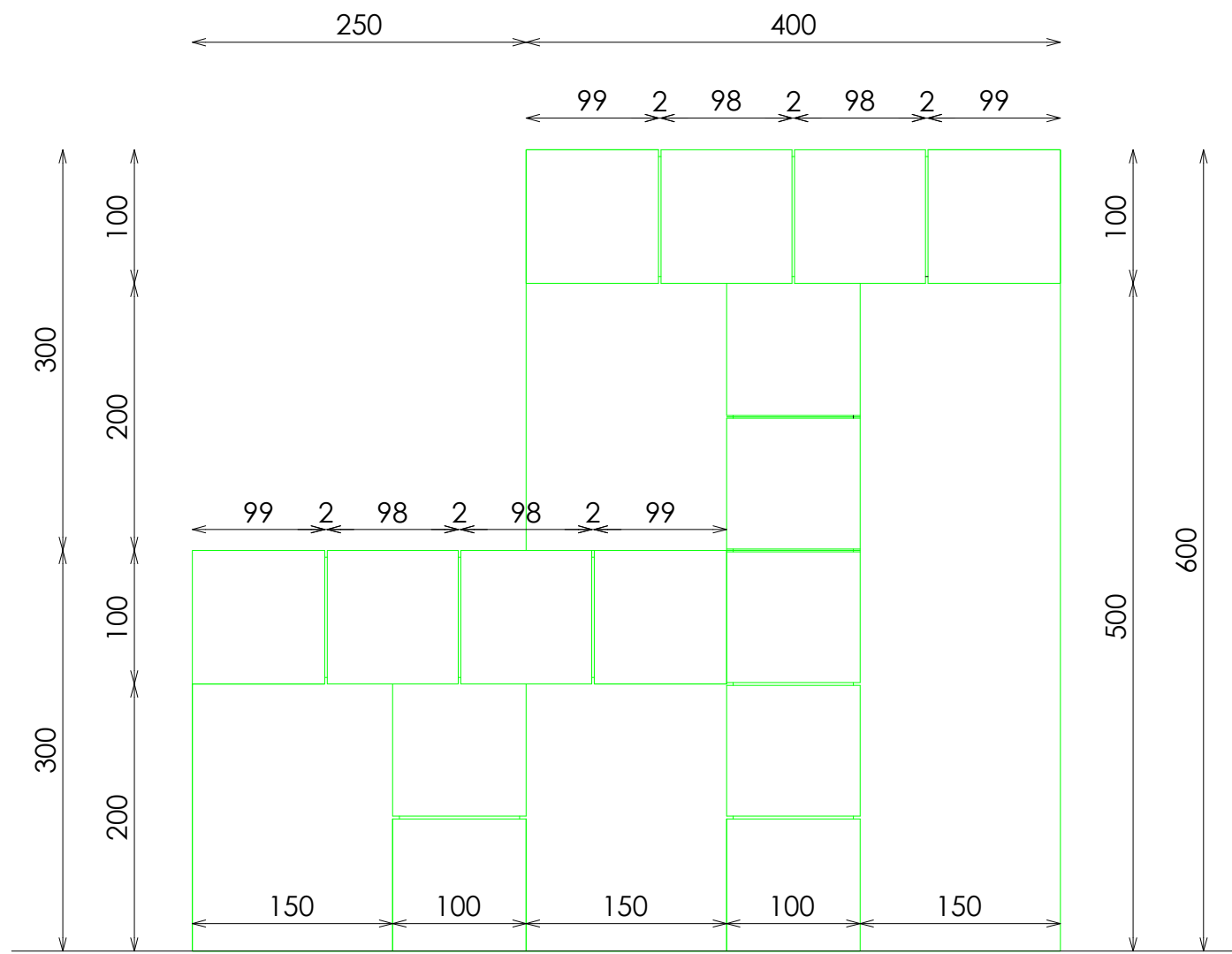
ALZADO
