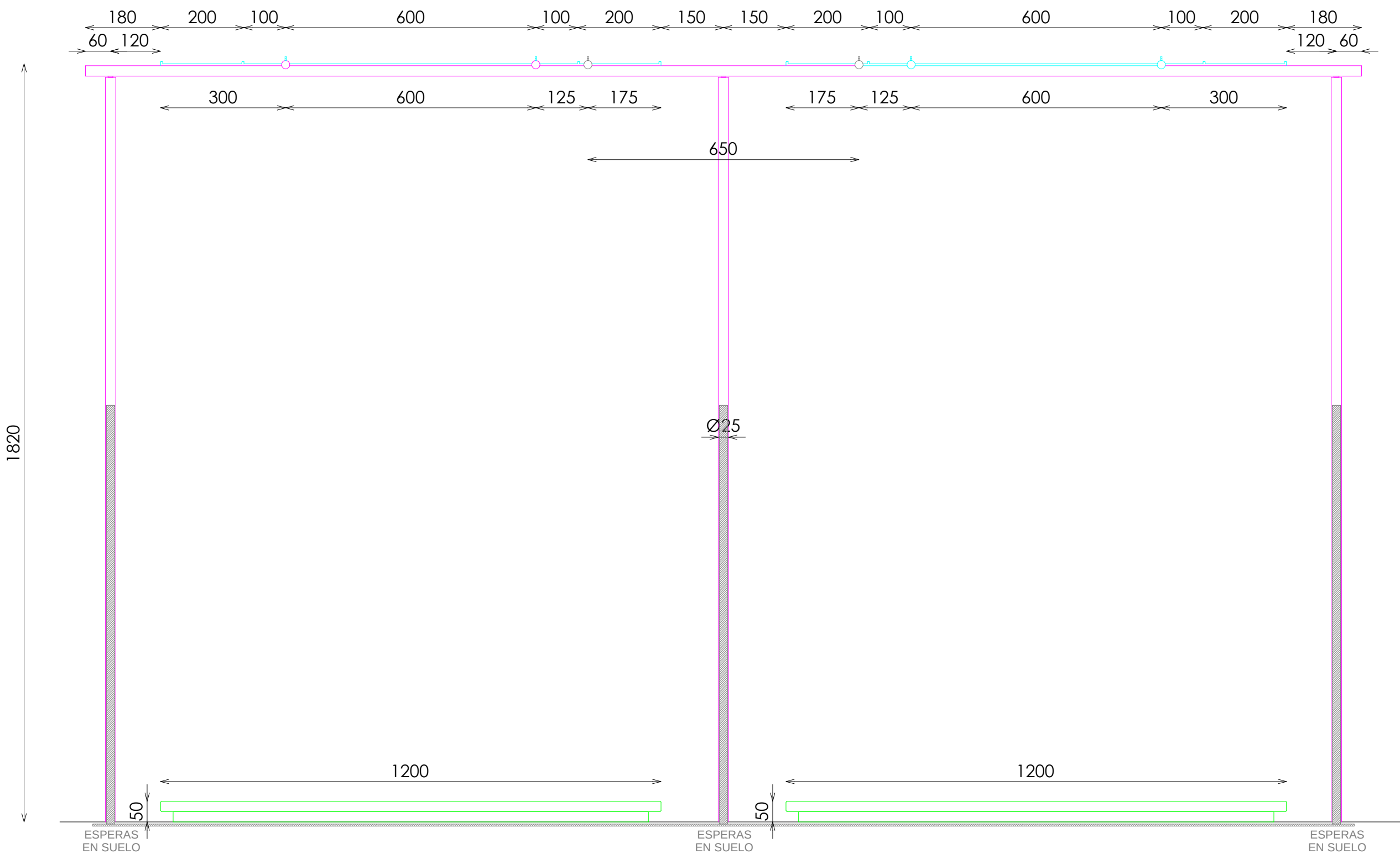
ALZADO FRONTAL
