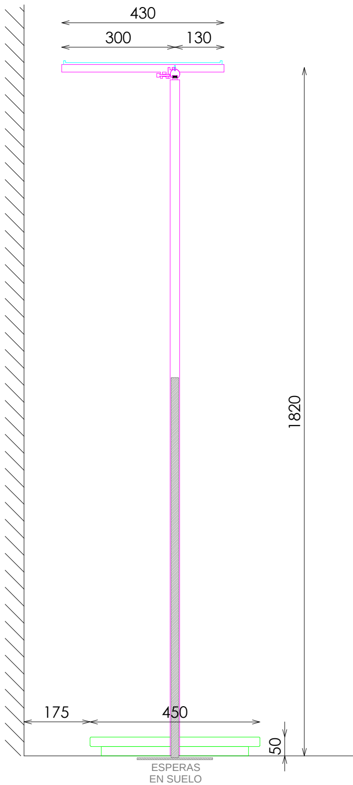
SECCIÓN
