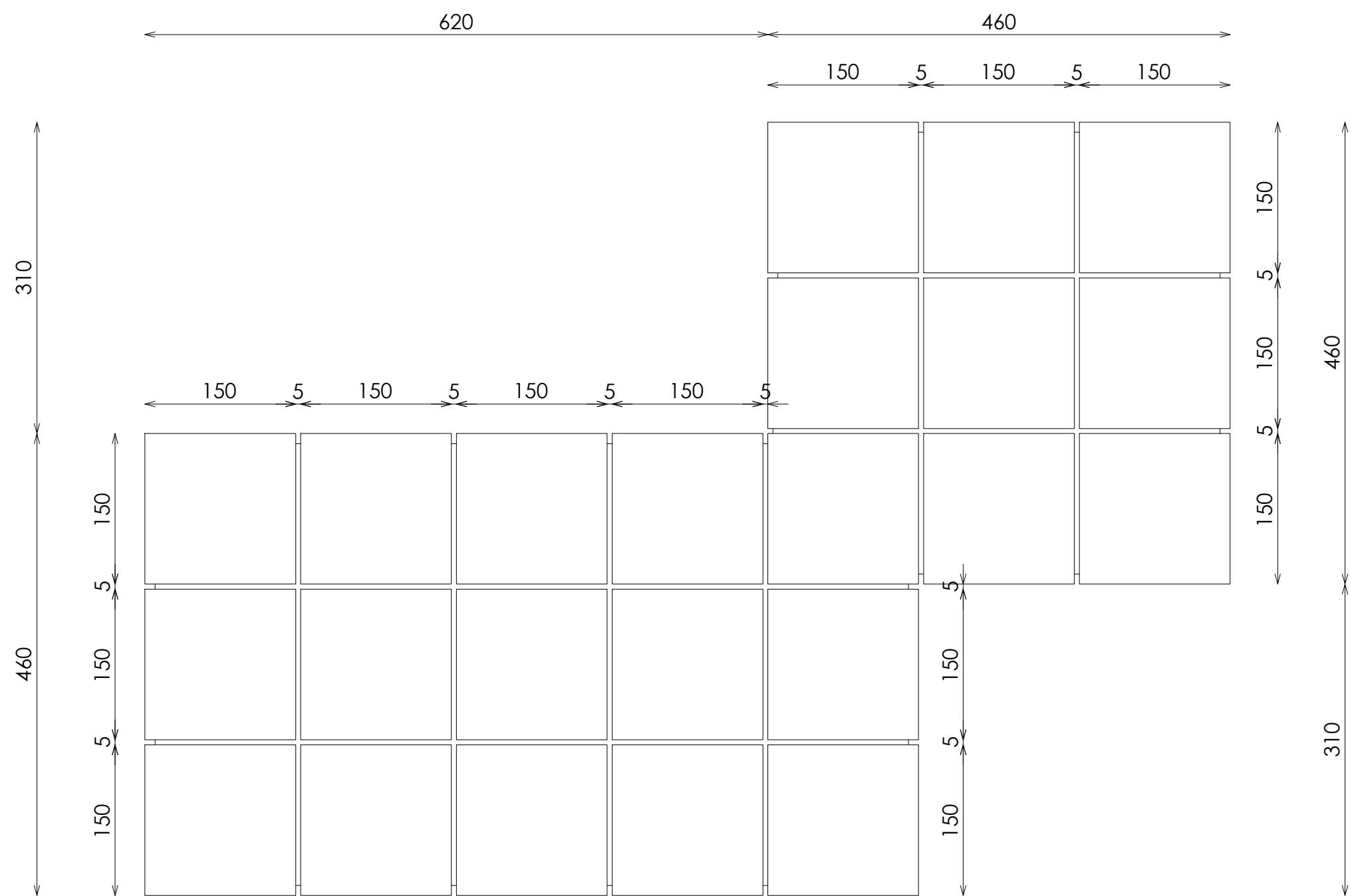
PLANTA
