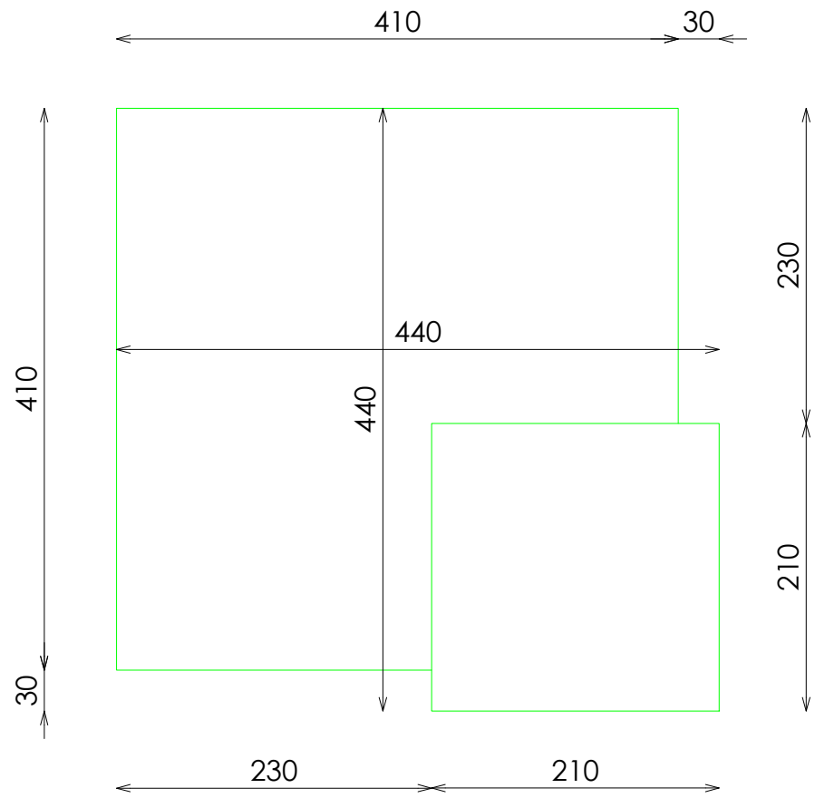
PLANTA
