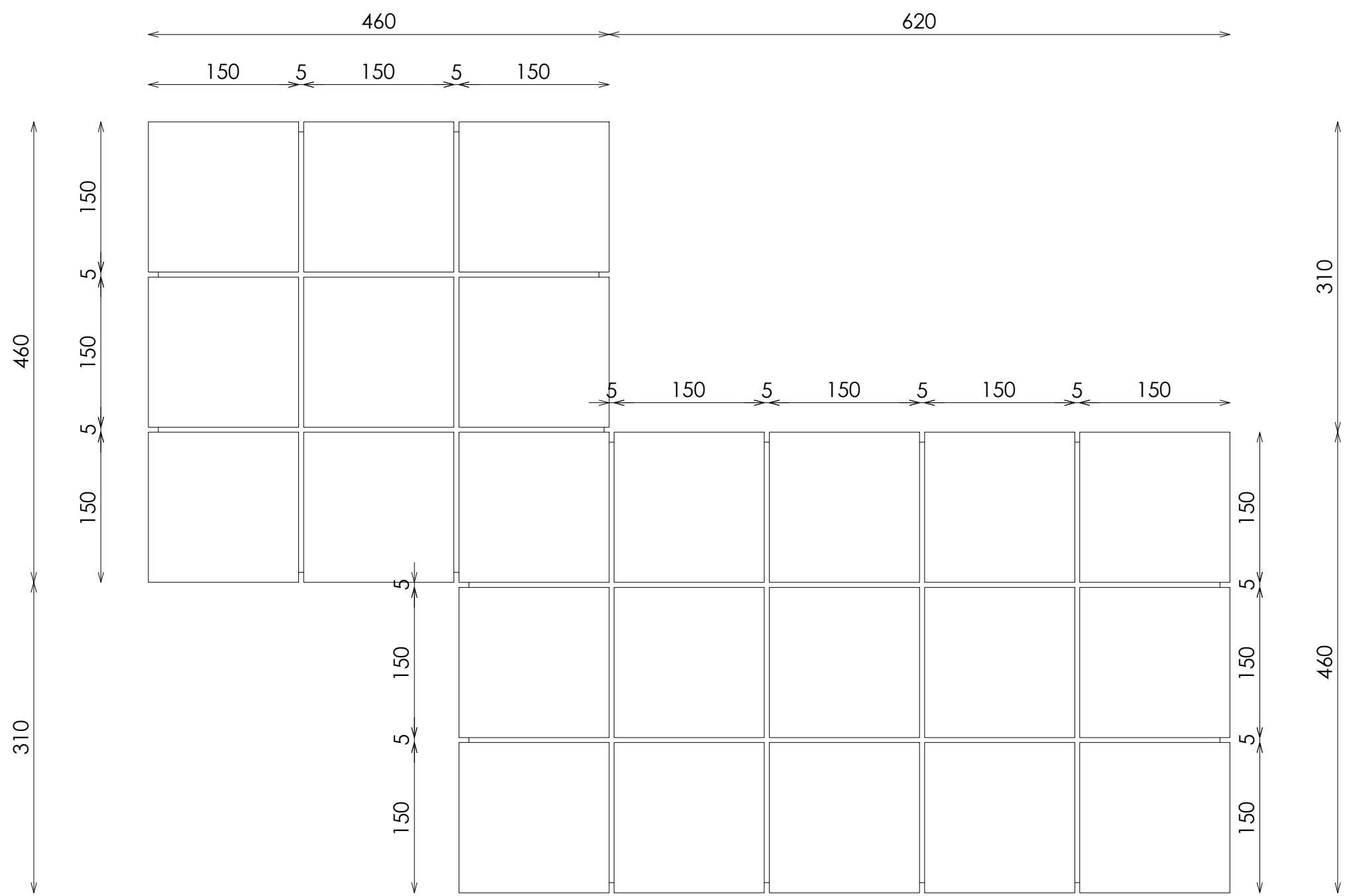
PLANTA
