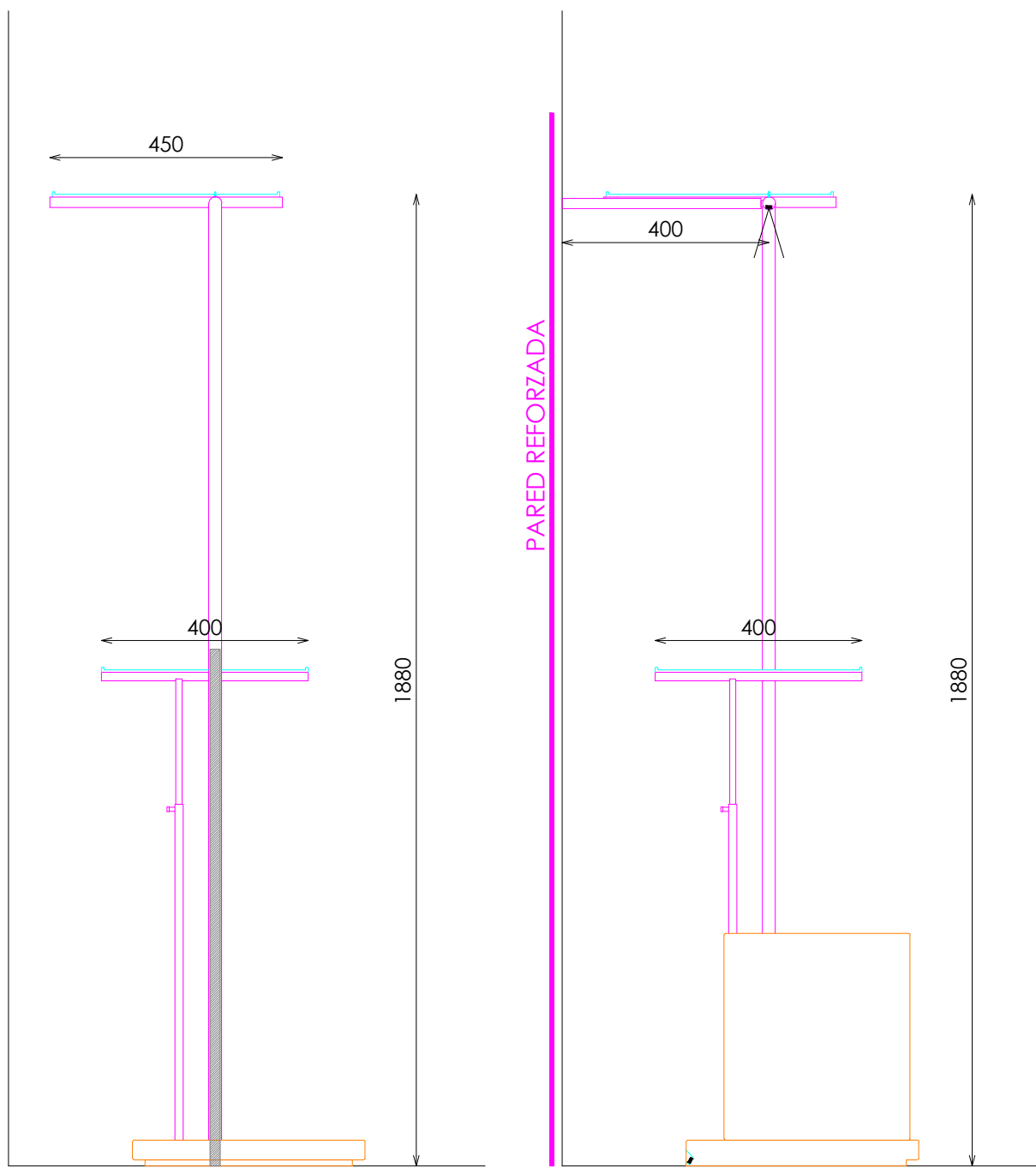
ALZADO LATERAL
