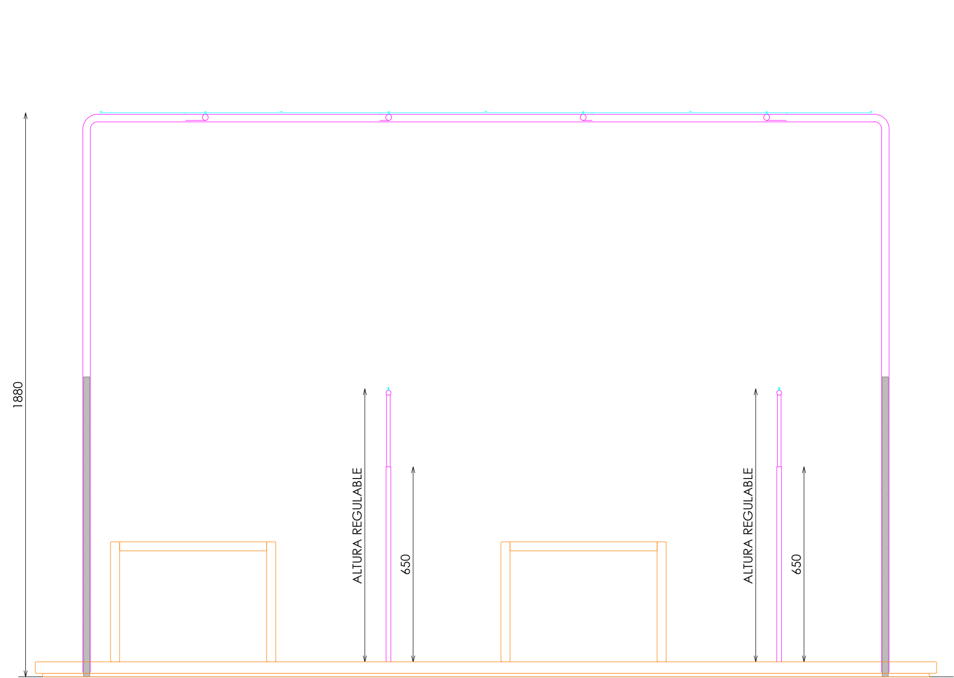
ALZADO FRONTAL
