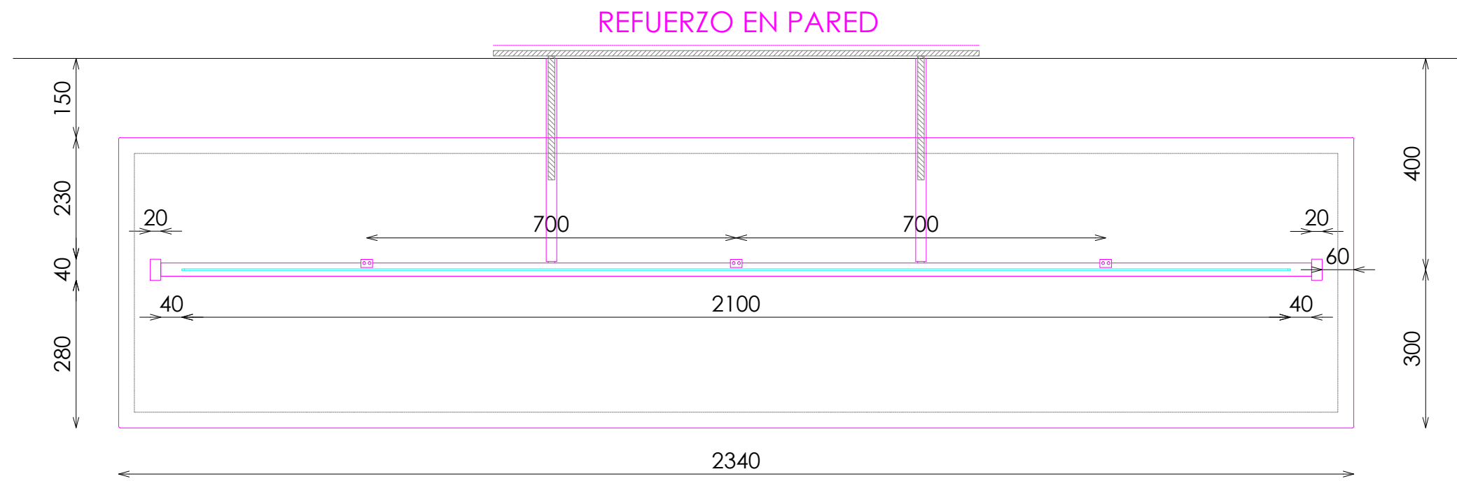
PLANTA
