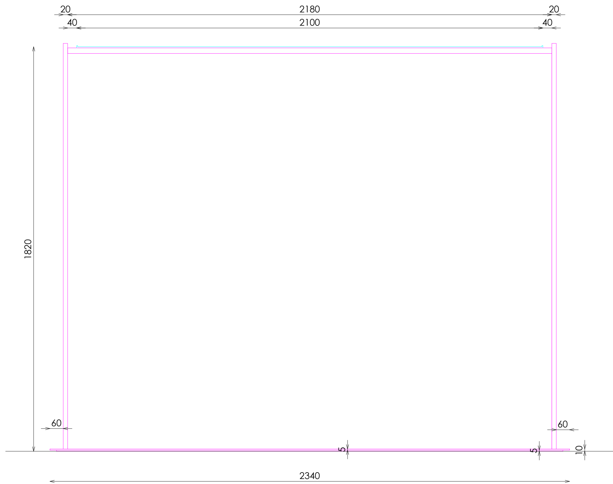
ALZADO SECCIONADO
