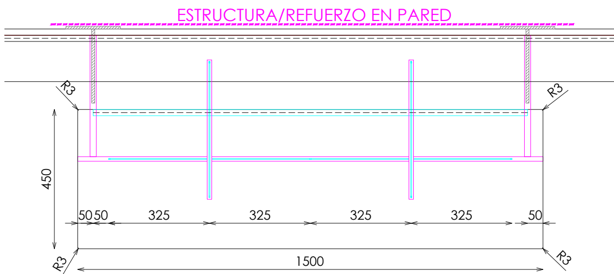
PLANTA
