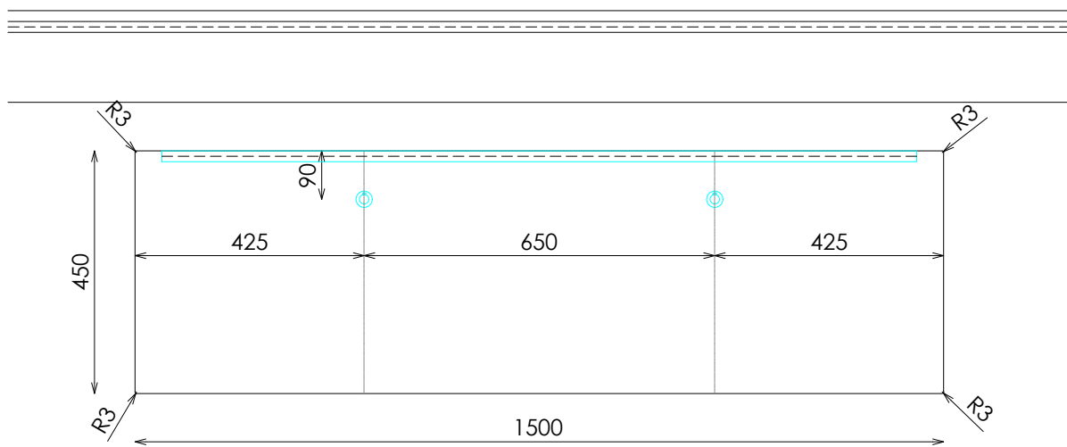
PLANTA (POSICIONES COLGADORES AUXILIARES)
