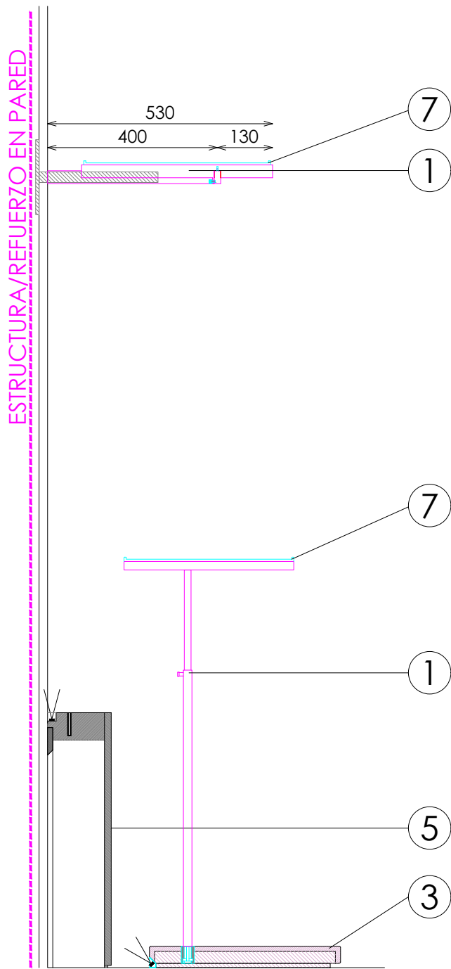
SECCIÓN
