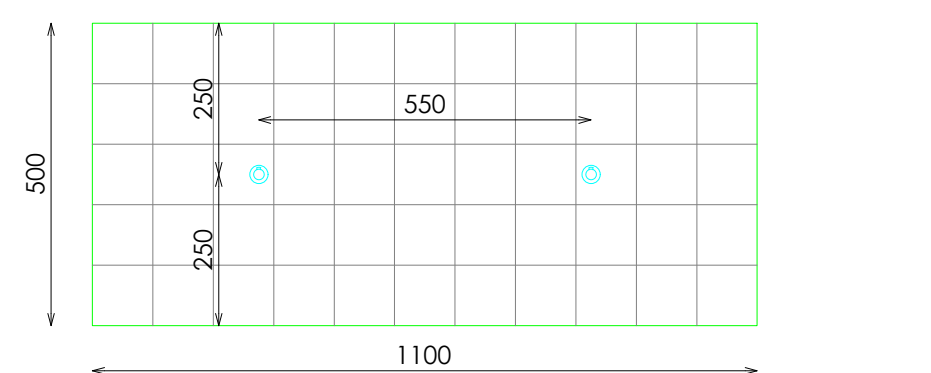
PLANTA (POSICIONES COLGADORES AUXILIARES)
