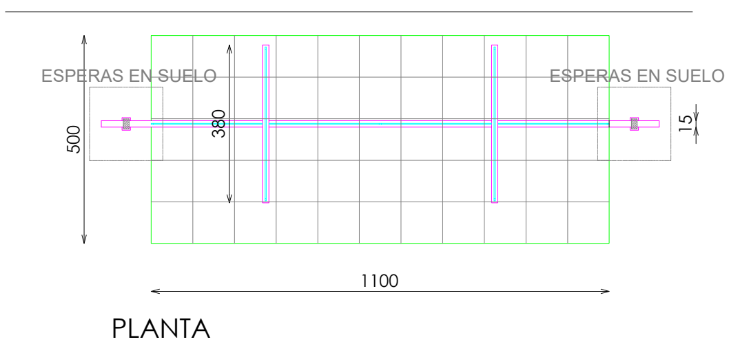
PLANTA
