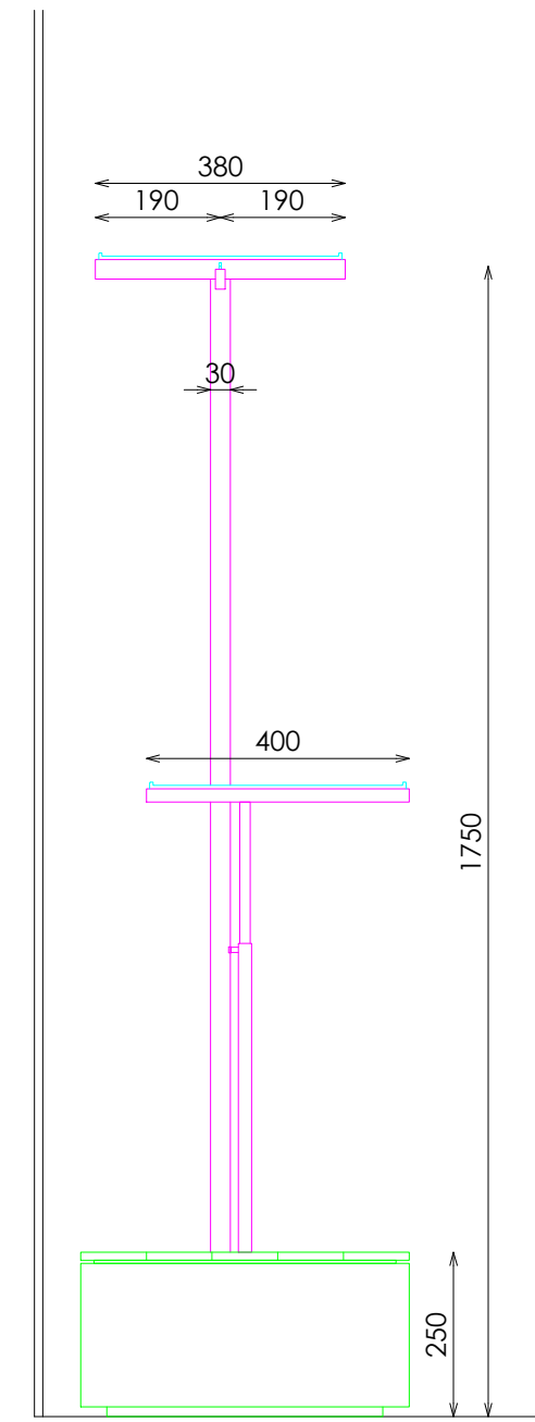
SECCIÓN
