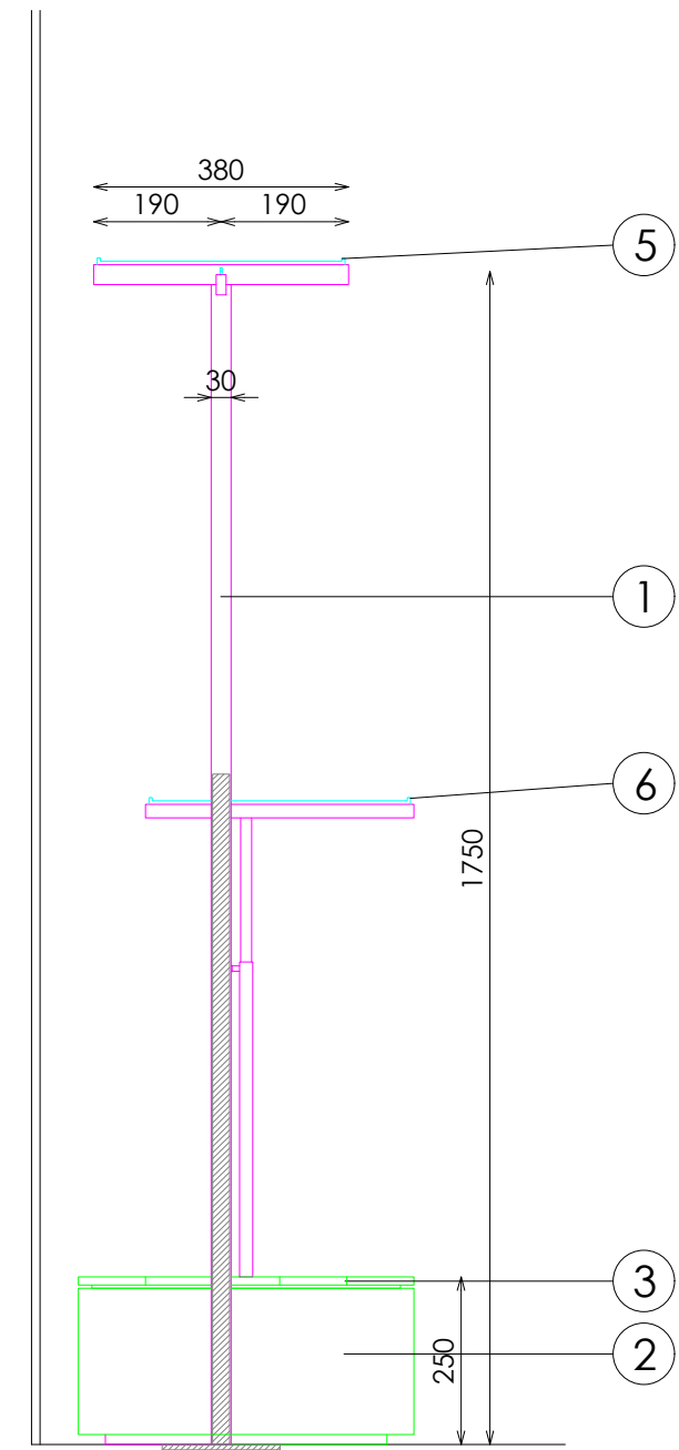
ALZADO LATERAL
