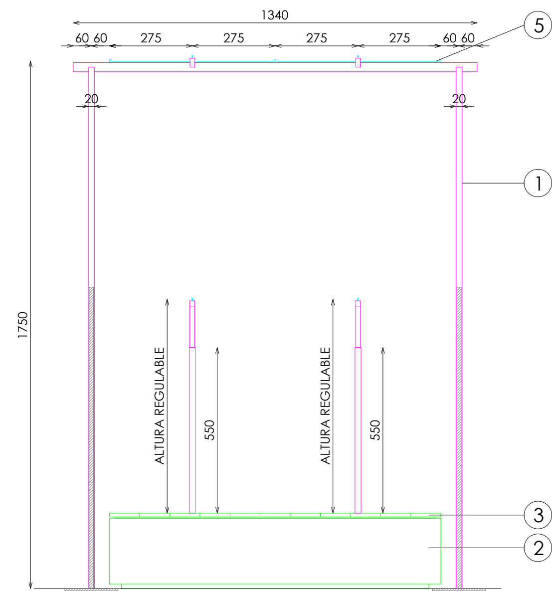
ALZADO FRONTAL
