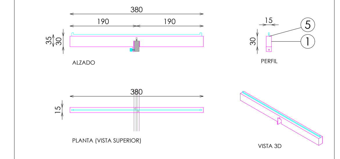
DETALLE A
