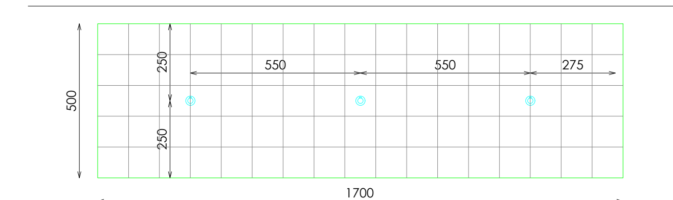
PLANTA (POSICIONES COLGADORES AUXILIARES)
