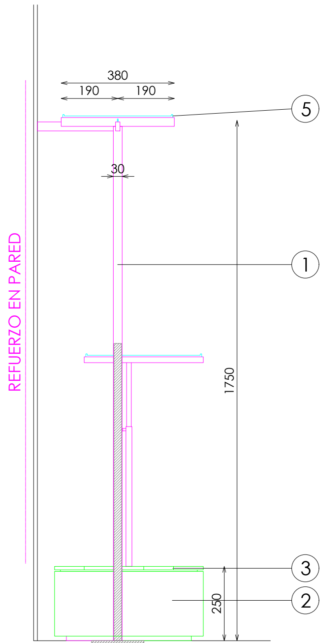
ALZADO LATERAL
