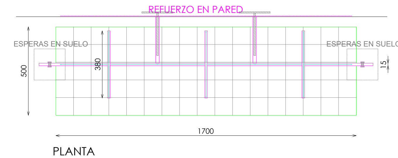
PLANTA
