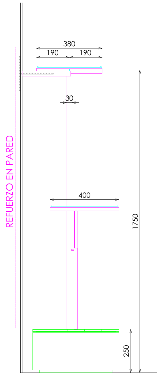
SECCIÓN
