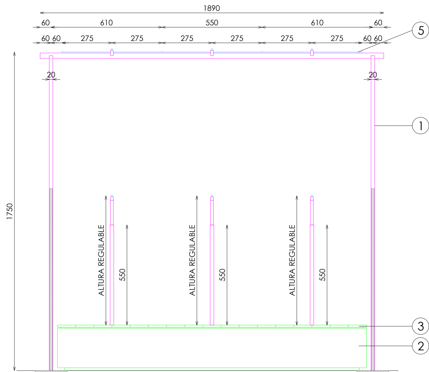
ALZADO FRONTAL
