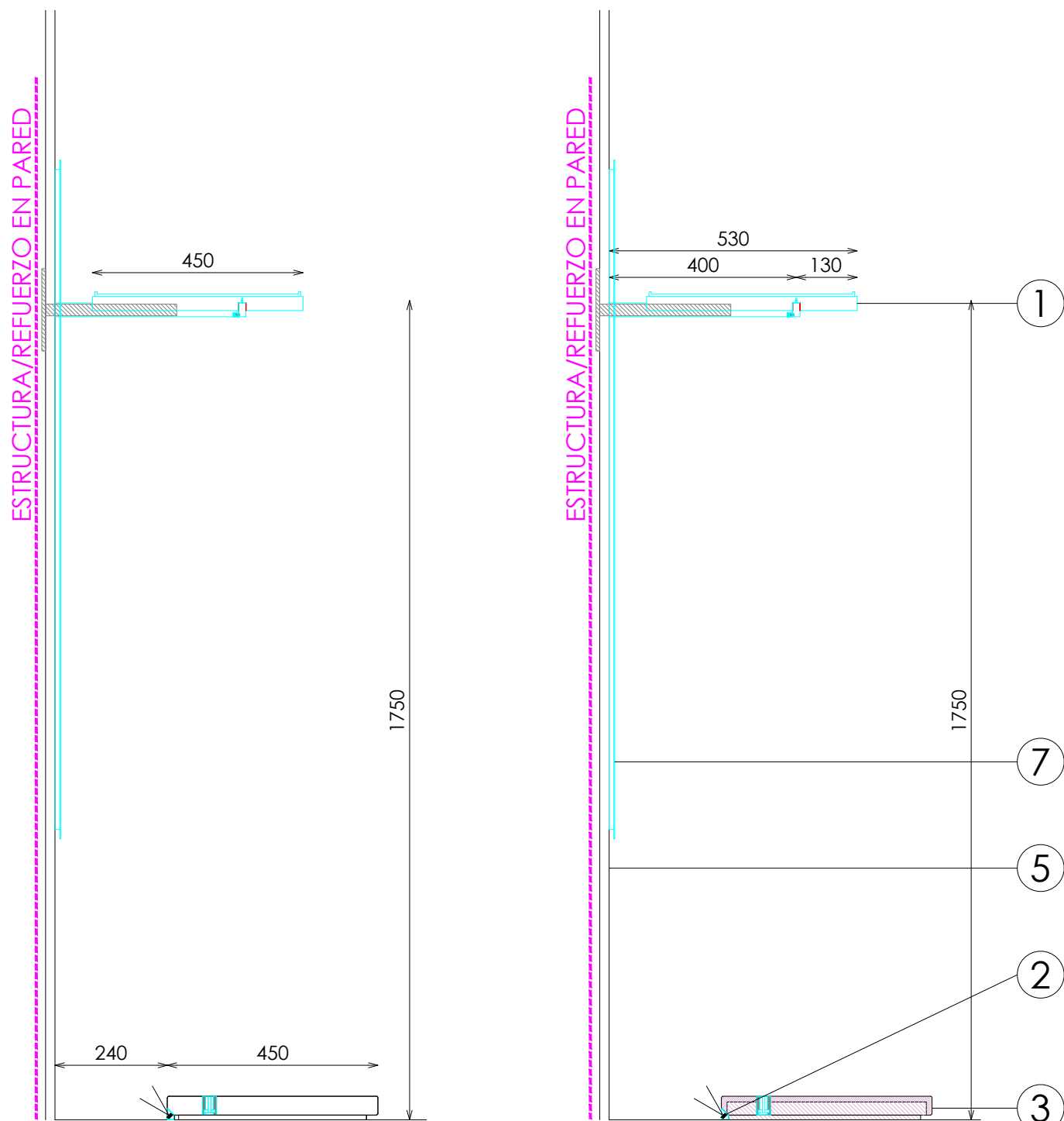
PERFIL
