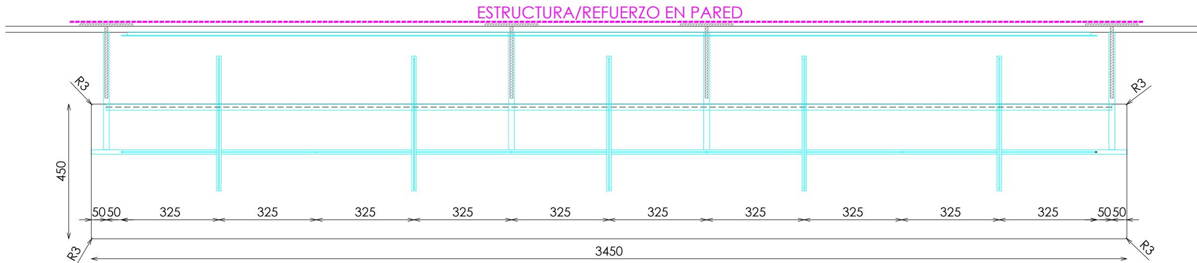
PLANTA
