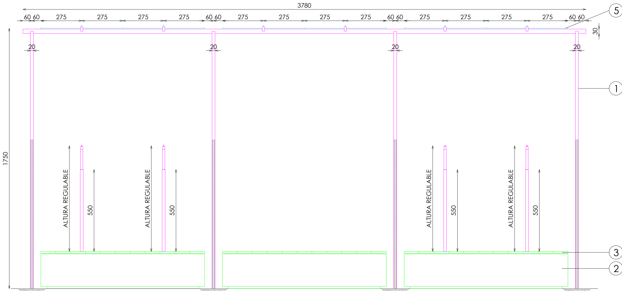
ALZADO FRONTAL
