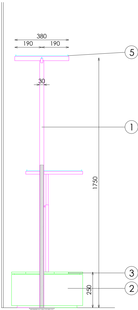
ALZADO LATERAL
