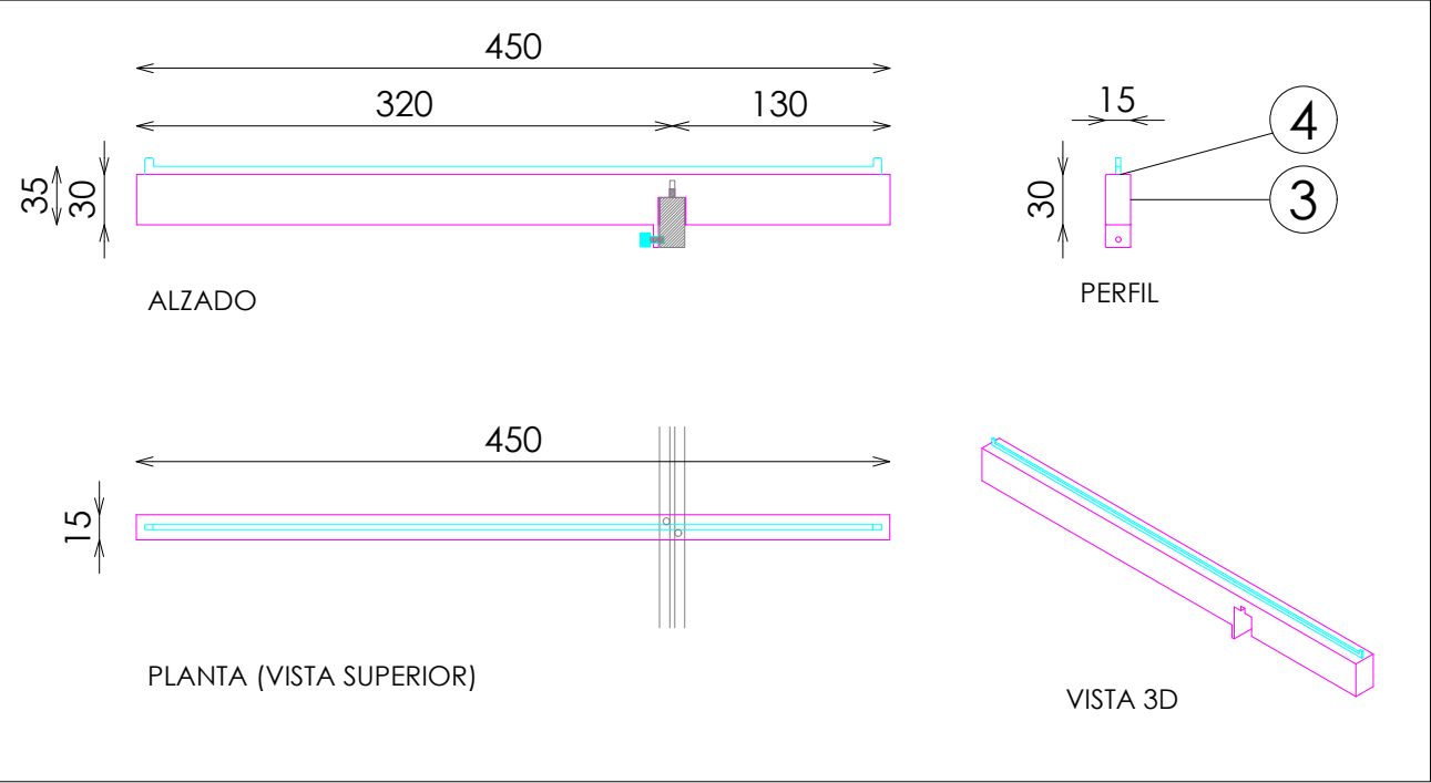
DETALLE FRONTALES EXTRAIBLES (TUBO MACIZO)
