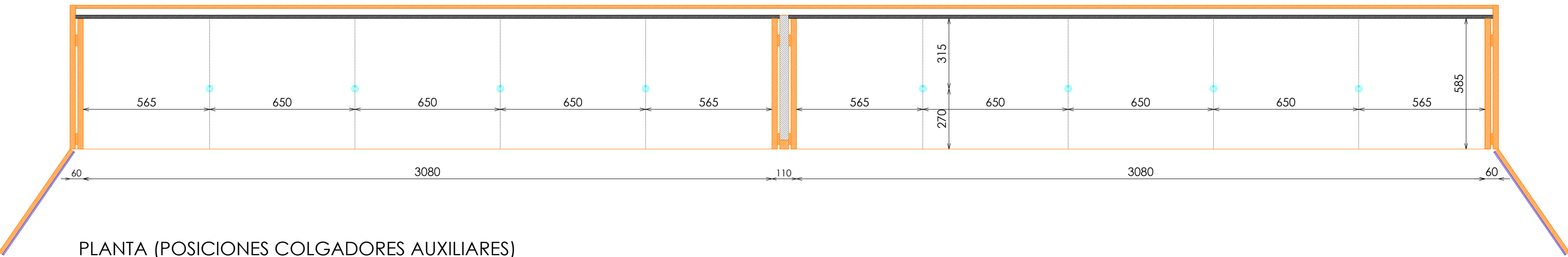
PLANTA (POSICIONES COLGADORES AUXILIARES)
