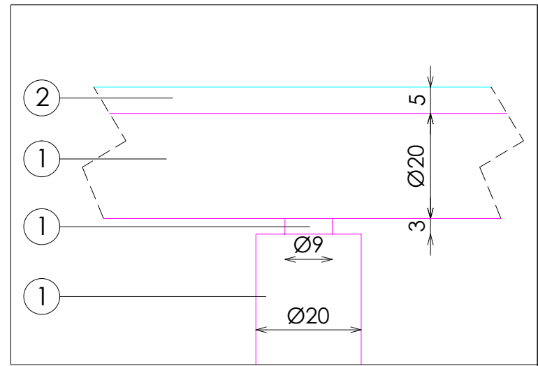
DETALLE B
