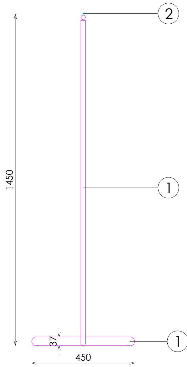
PERFIL
