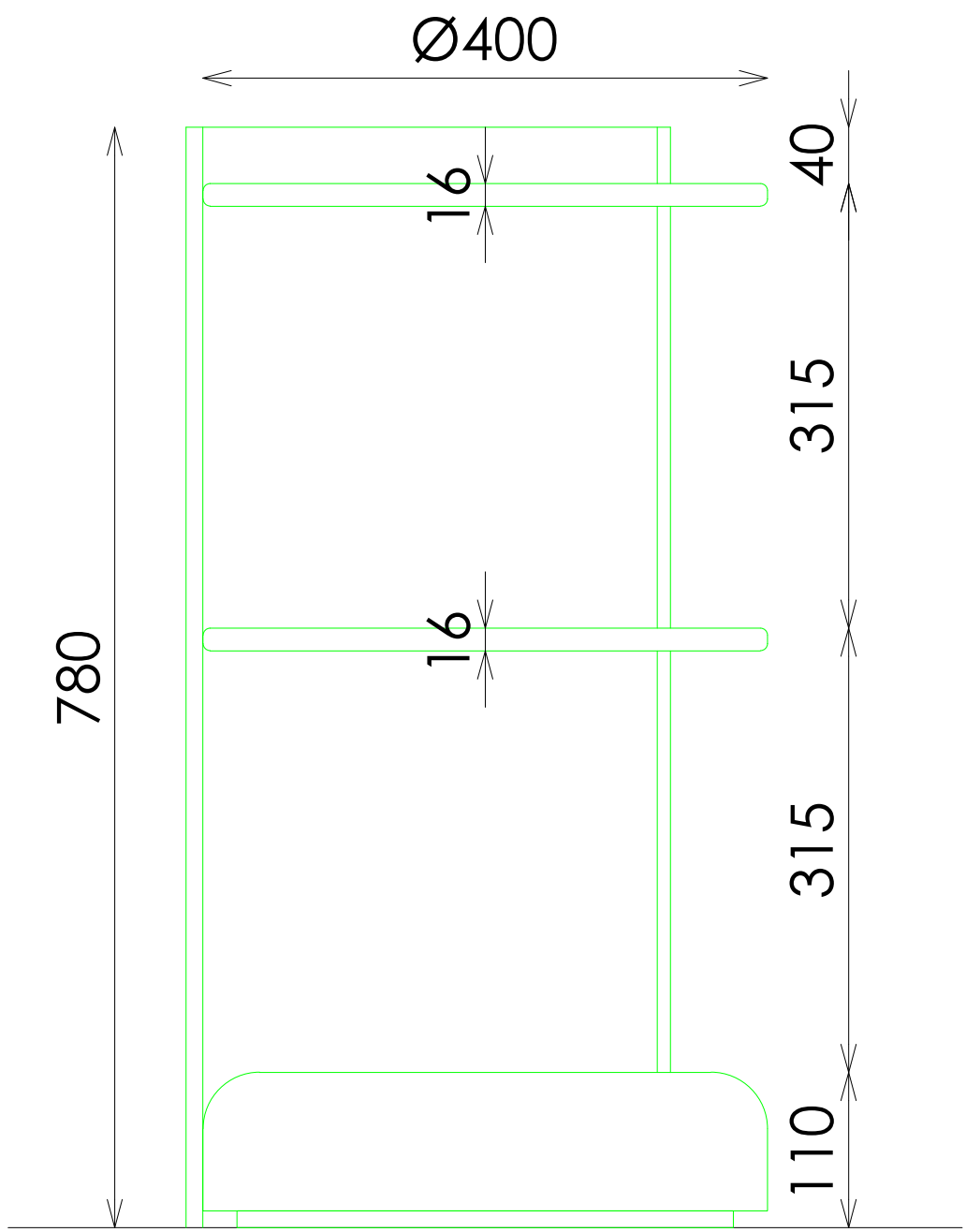
ALZADO
