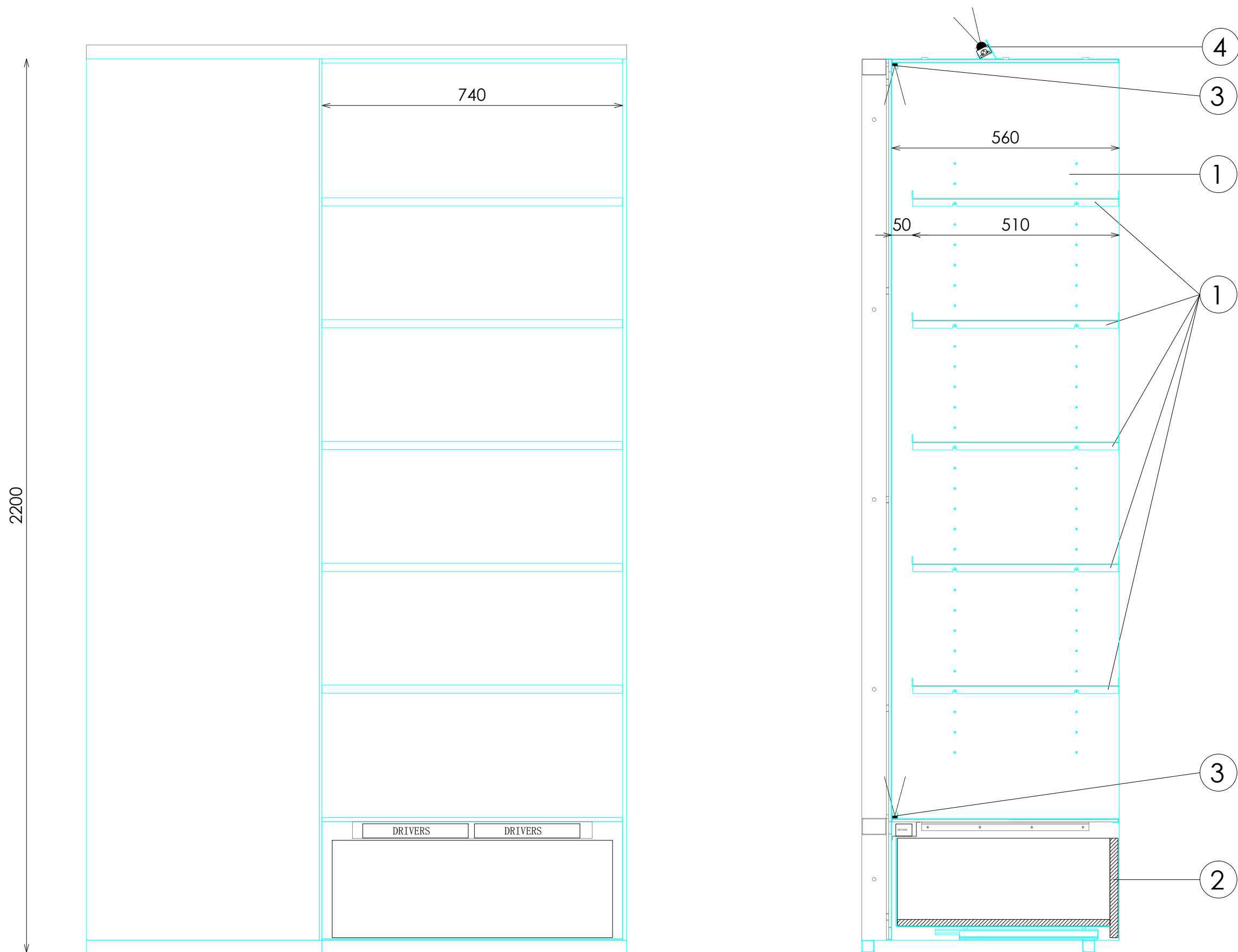
ALZADO
