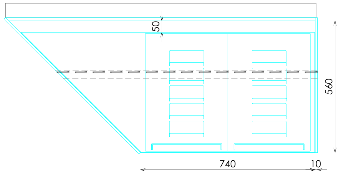
PLANTA ESTANTES
