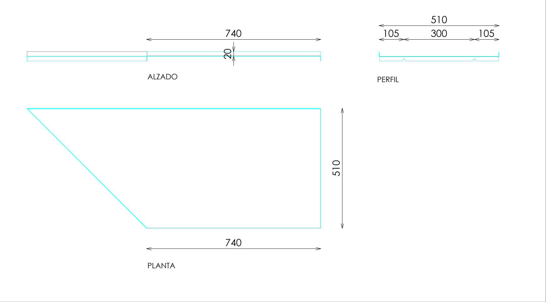
DOTACION ESTANTES
