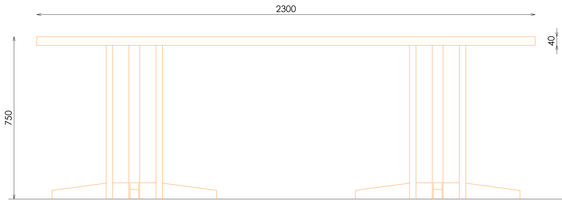
ALZADO FRONTAL
