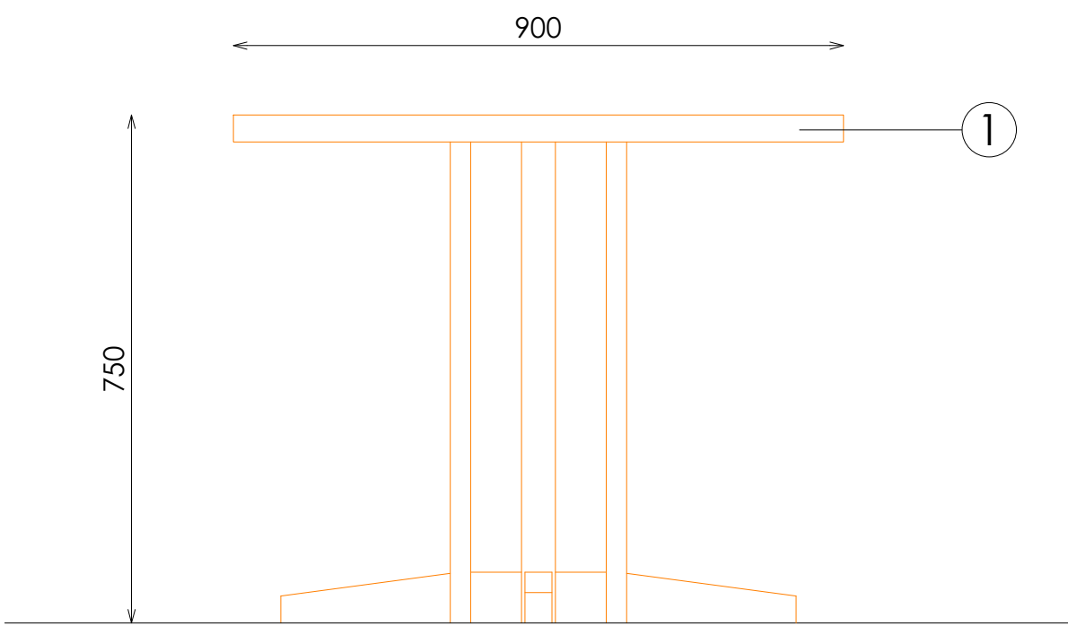
ALZADO LATERAL
