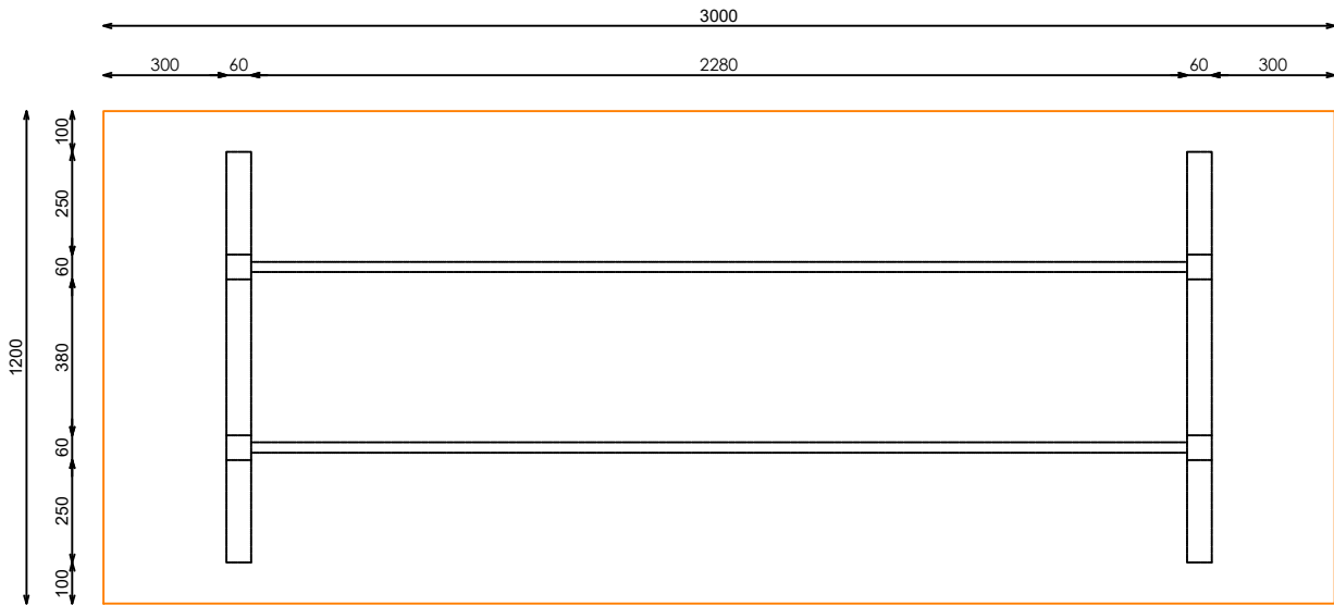
PLANTA SECCIONADA
