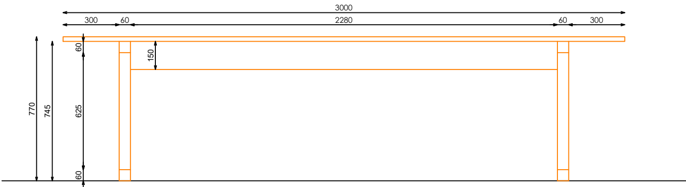
ALZADO FRONTAL
