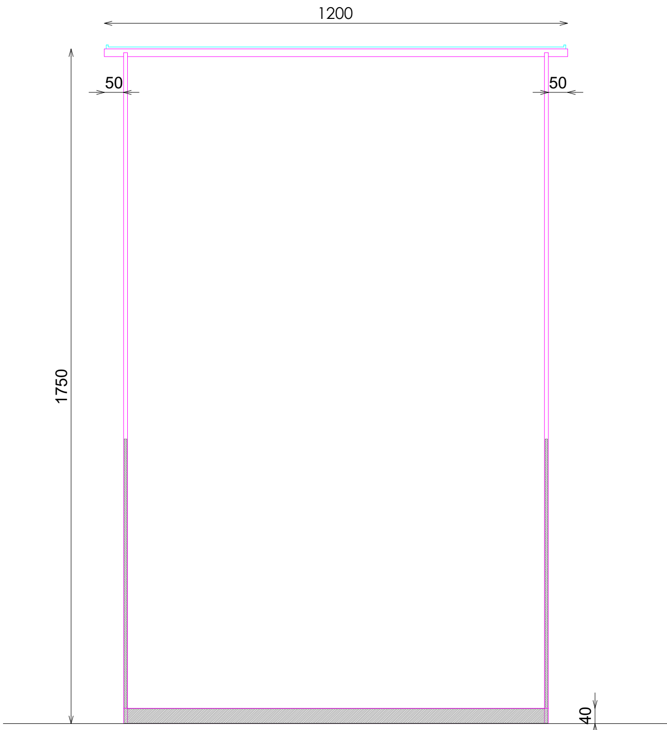
ALZADO
