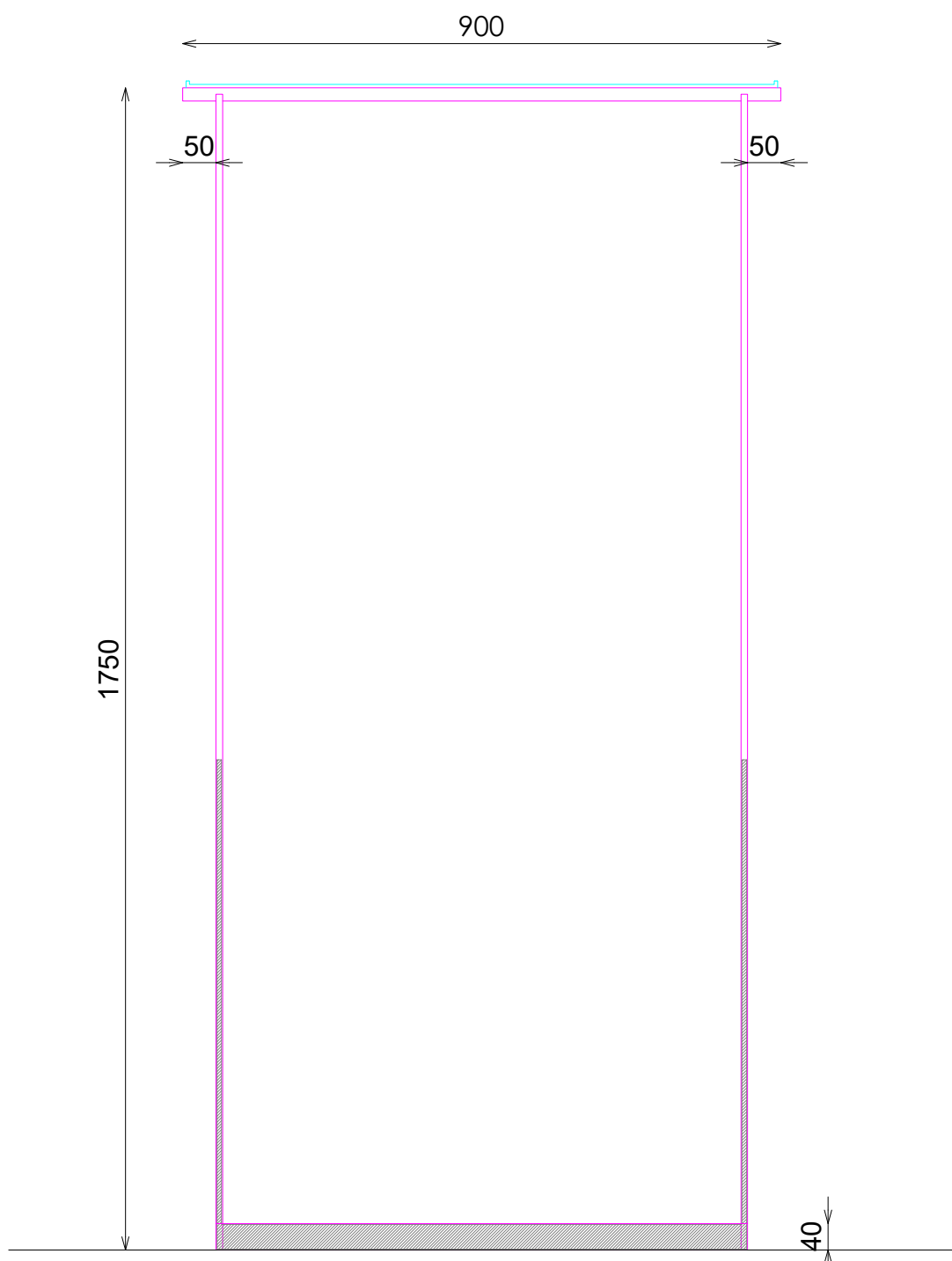
ALZADO
