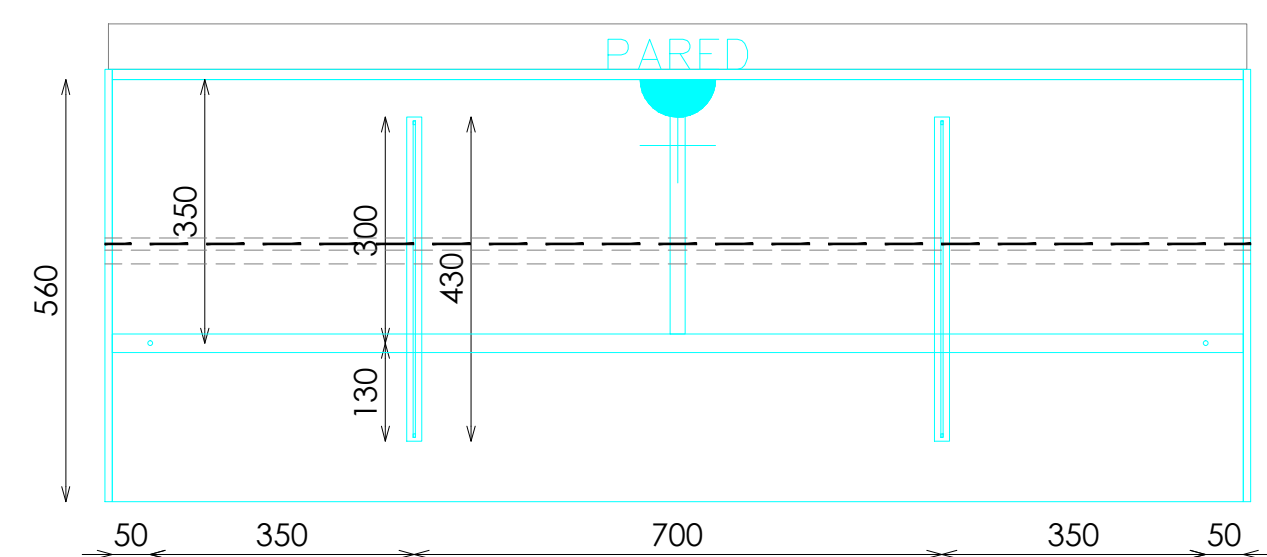
PLANTA BARRA
