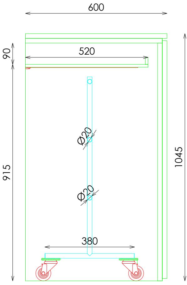
SECCION BURRO
