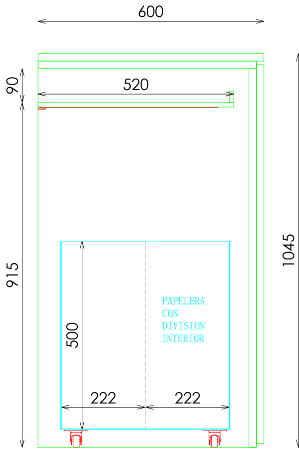
SECCION PAPELERA
