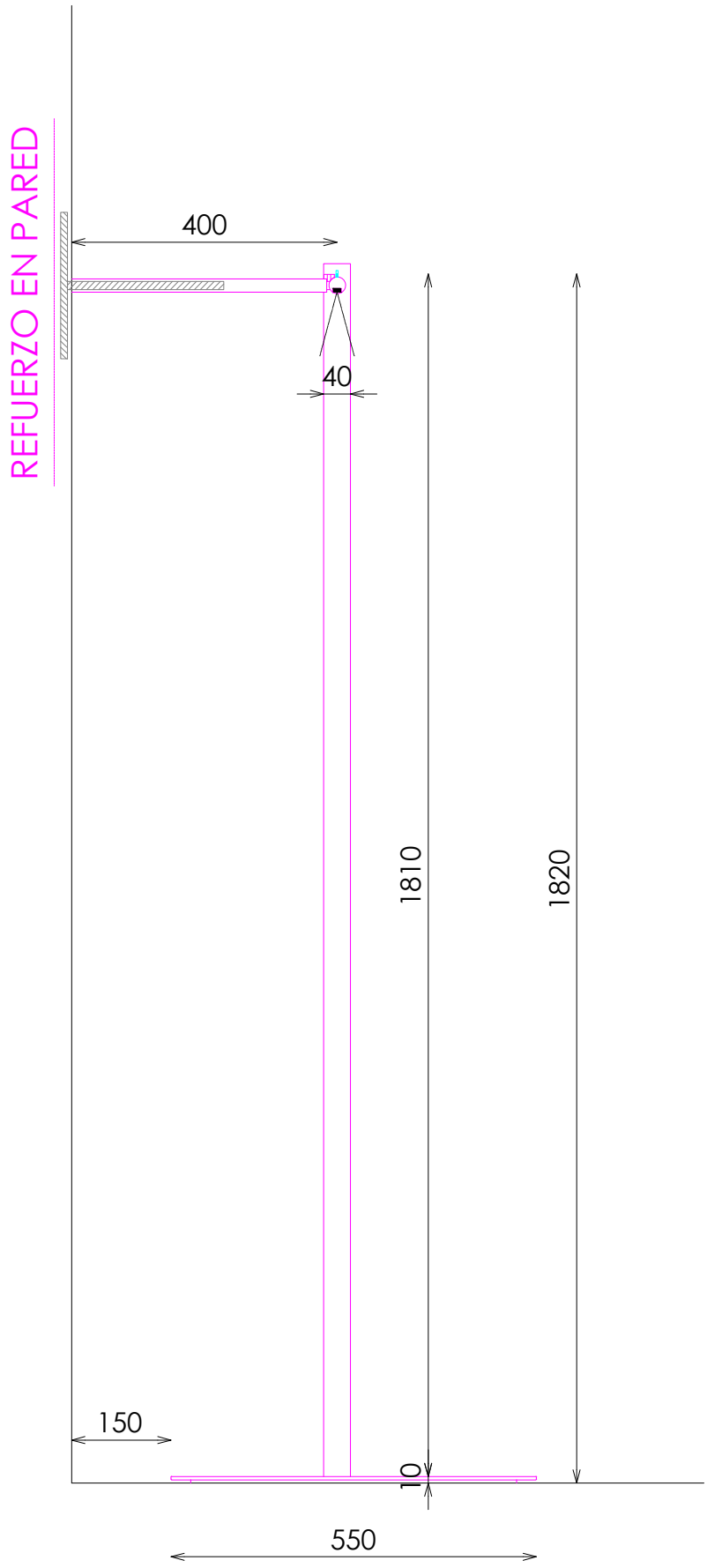
PERFIL SECCIONADO
