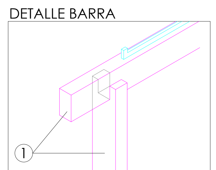
DETALLE BARRA
