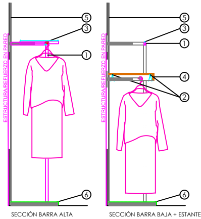
SECCIÓN BARRA ALTA
