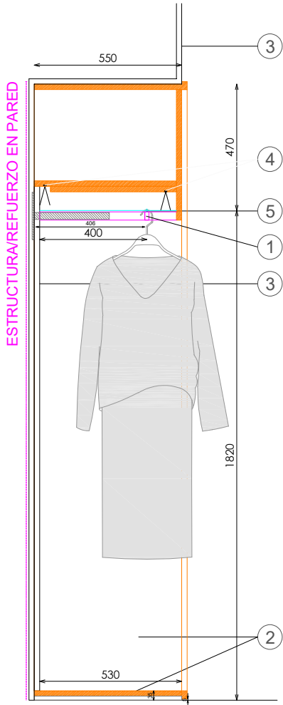
SECCIÓN
