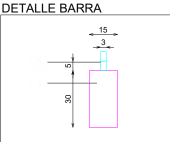
DETALLE BARRA
