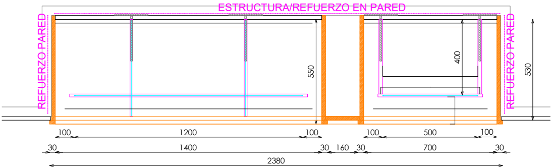
PLANTA
