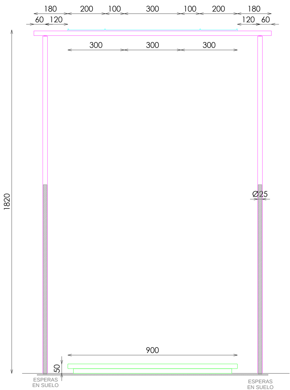
ALZADO FRONTAL
