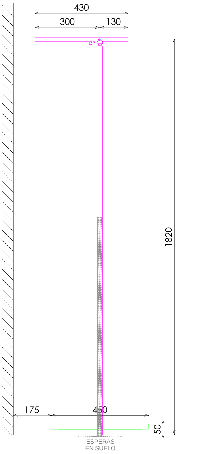
SECCIÓN
