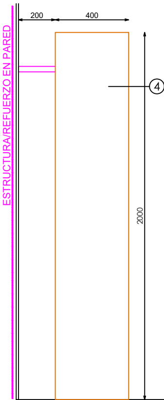
ALZADO LATERAL
