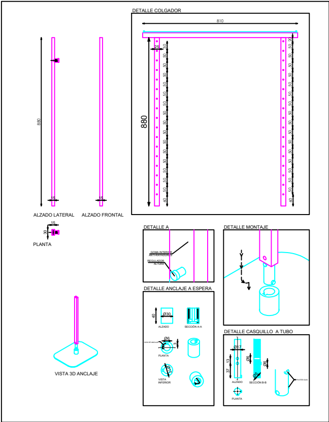
DETALLE COLGADOR INFERIOR EXTRAIBLE
