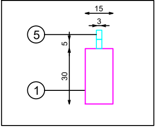
DETALLE BARRA
