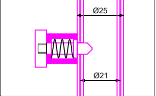
DETALLE SISTEMA ANCLAJE
